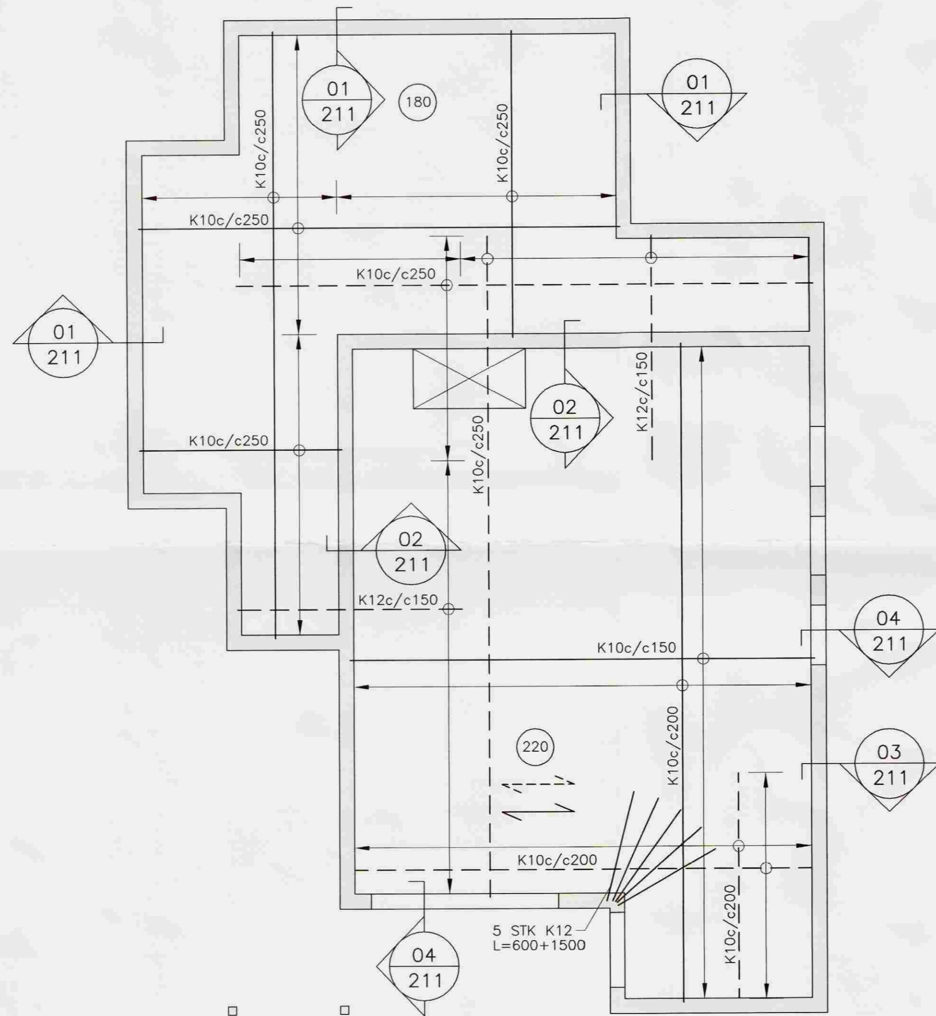
GRUNNMYND KJALLARA, 1:50
