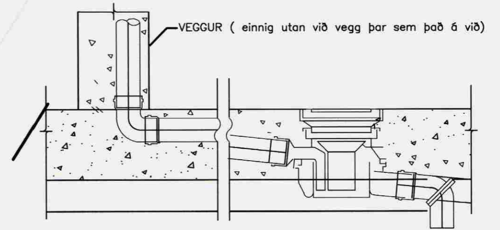
GÓLFNIDURFALL MED GEGNUMRENSLI, 1:5
