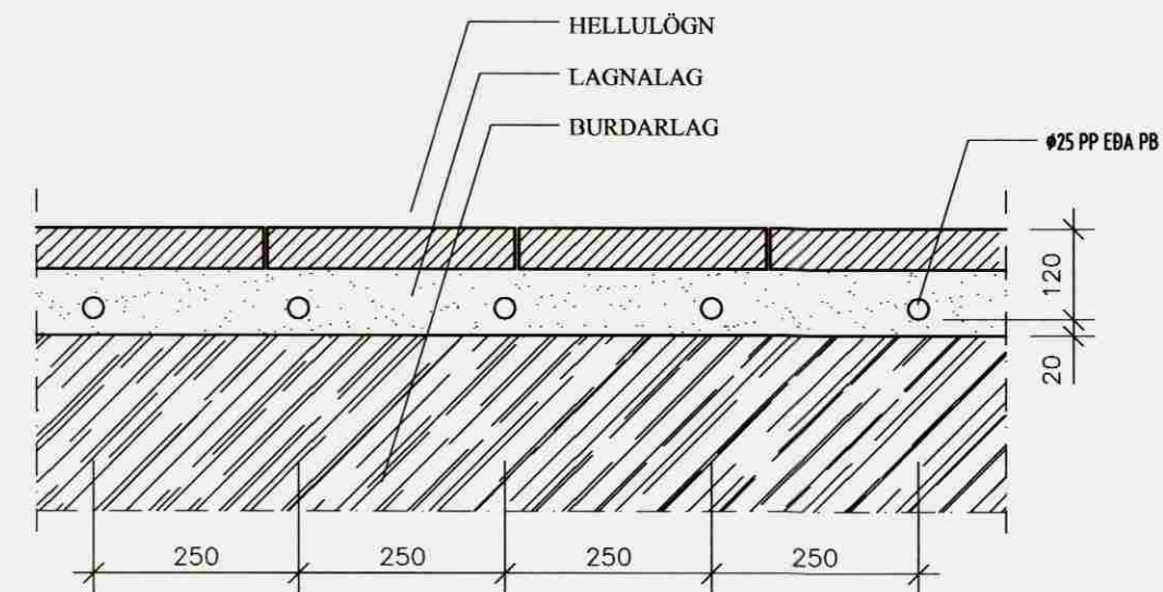
SNID Í SNJÓBRÆÐSLULÖGN UNDIR HELLUM, 1:10
