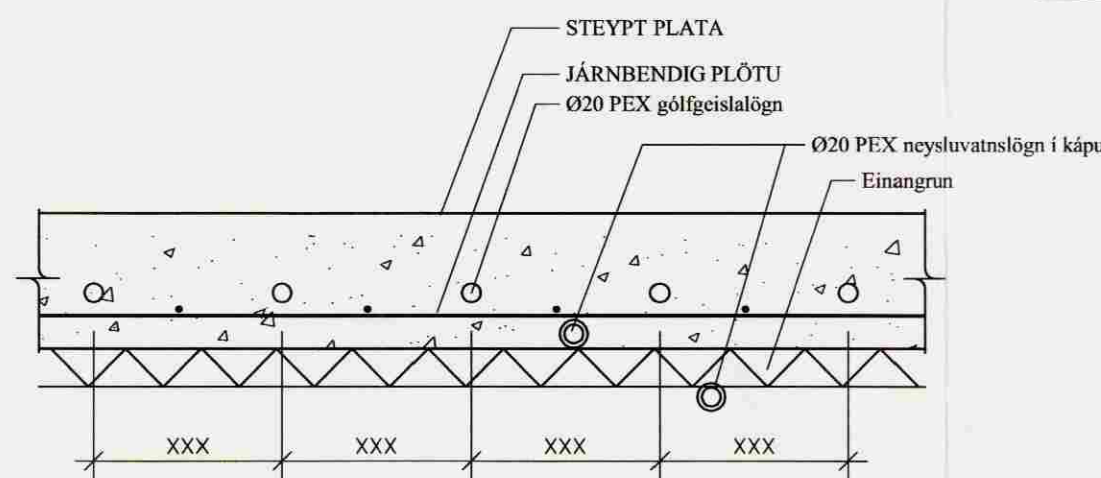
SNID Í GÓLFHITALÖGN, 1:10
