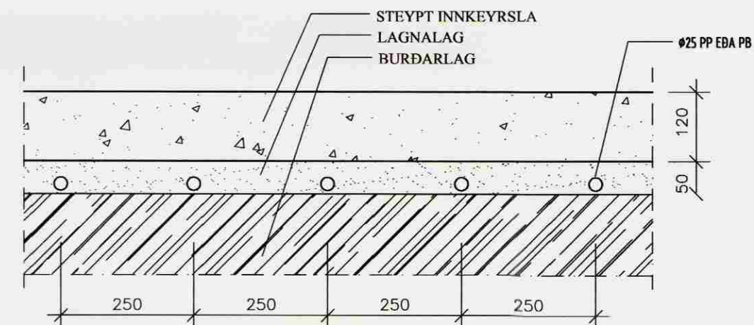
SNID Í SNJÓBRÆÐSLULÖGN UNDIR STEYPTU PLANI, 1:10
