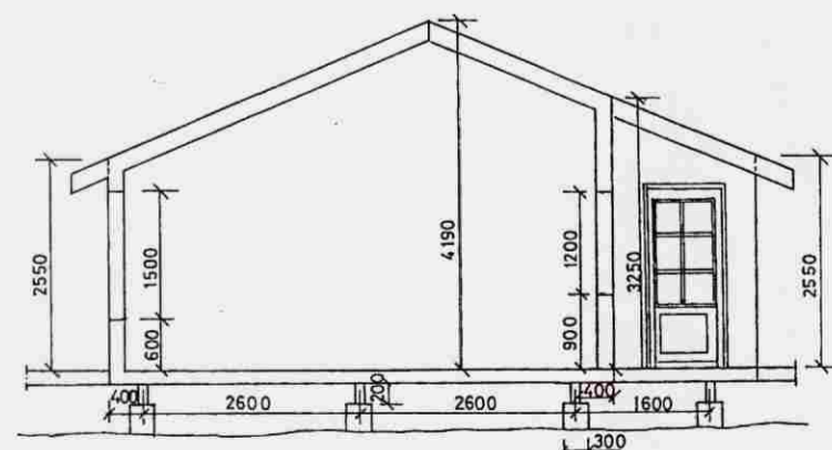
SNIÐ A-A 1: 100
