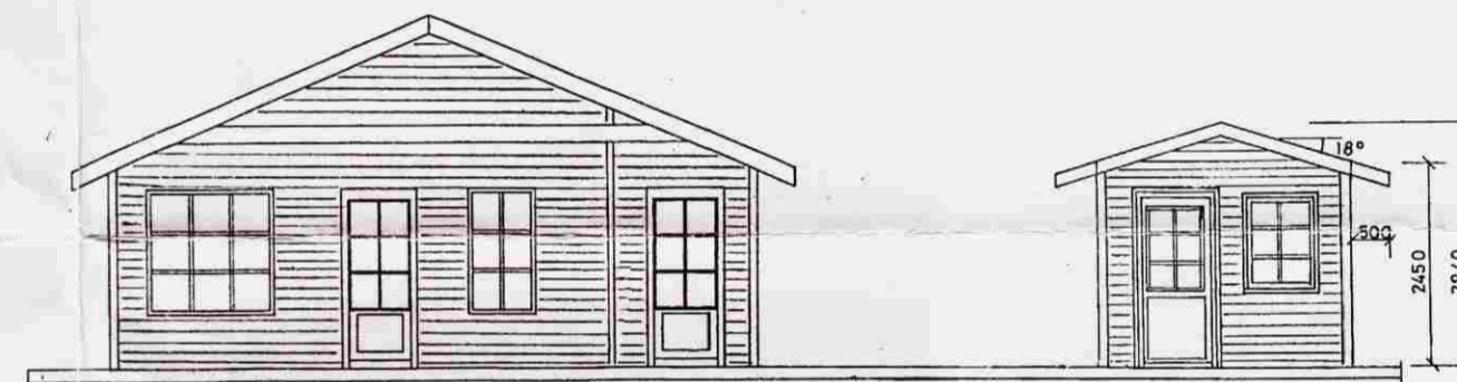
SUÐURHLIÐ 1: 100
