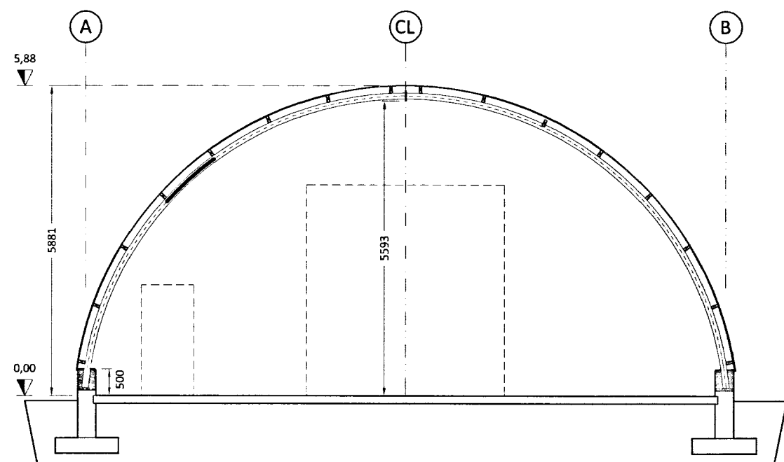
SNID A-A Mkv. 1:100
