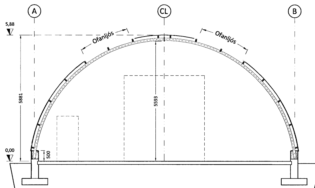
SNID B-B Mkv. 1:100
