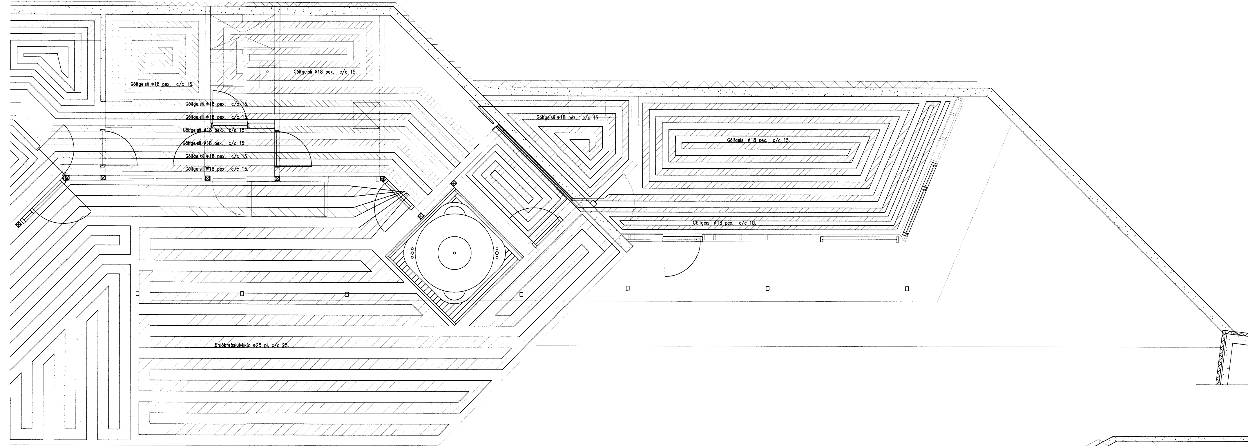
Hitalögn: Grunnmynd hæðar. 1:50.
