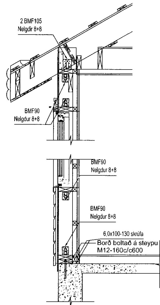
5 Veggssnið 1:20
