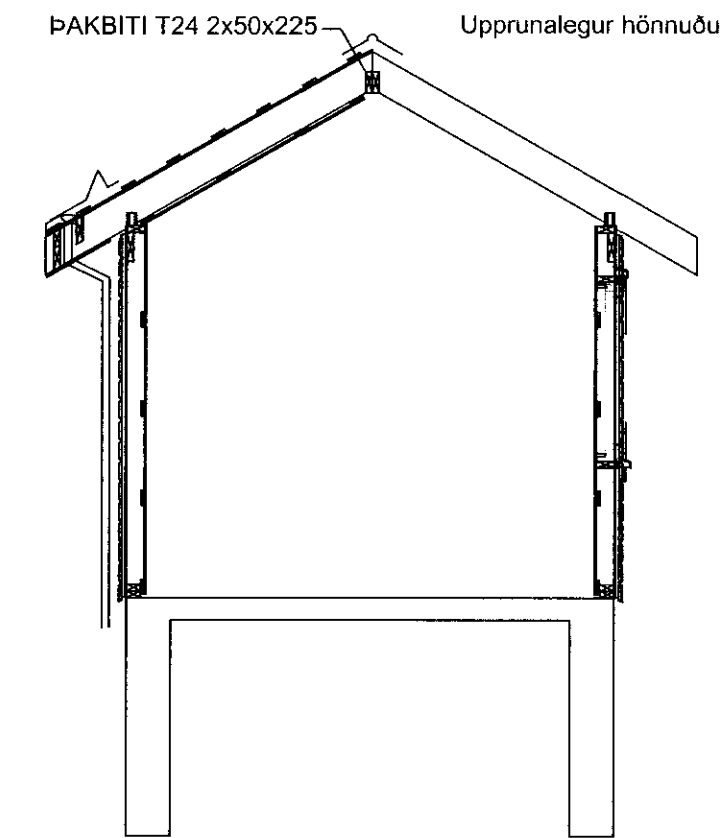
4 Snið 1:50
