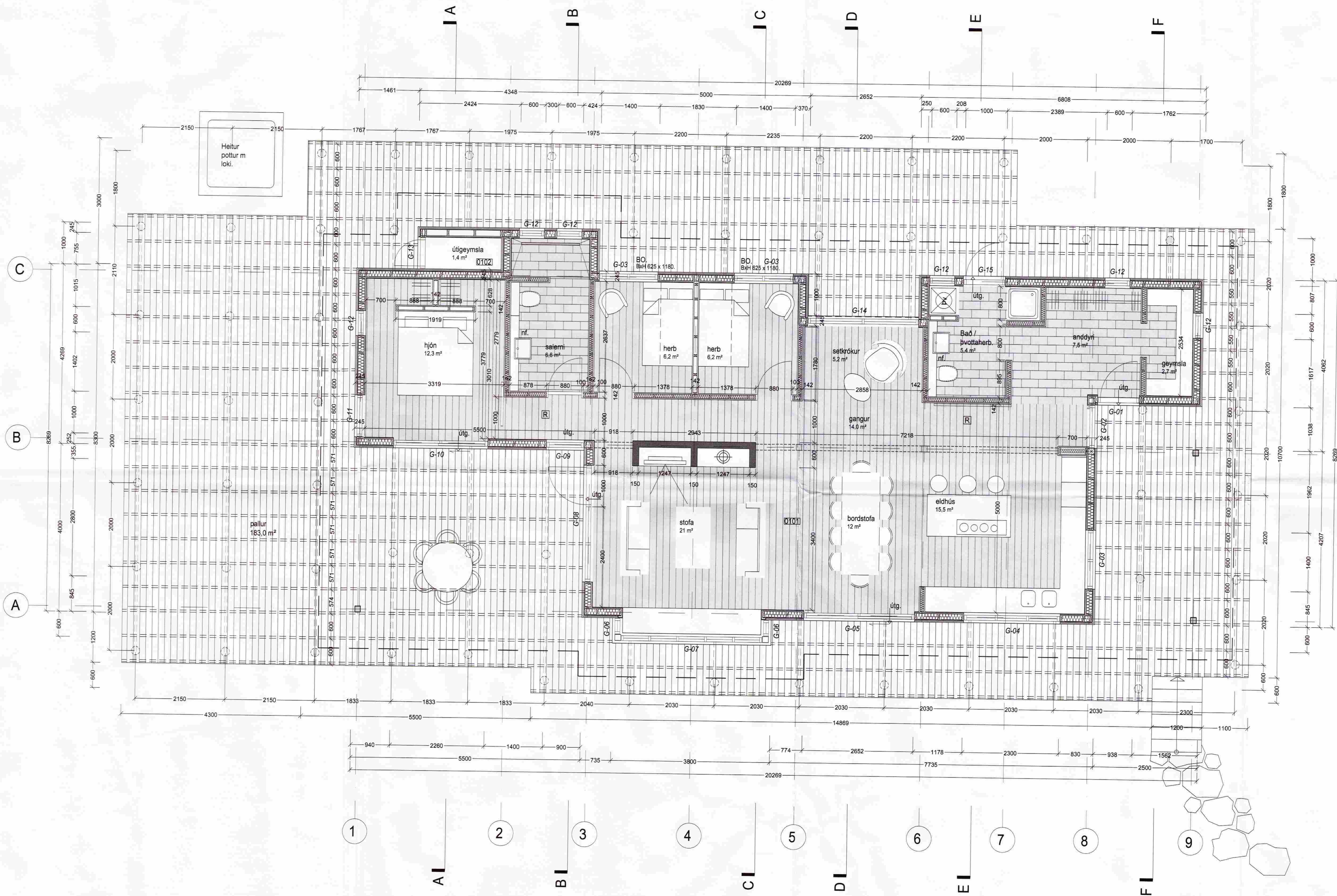
GRUNNMYND M 1:50
