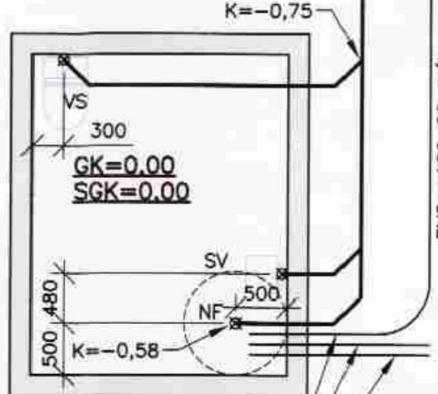
AFSTALL HITAVEITU PEH ø32 INNTAK HEITT NEYSLUVATN ø32 PEH | ø50 FÖDURRÖRI
