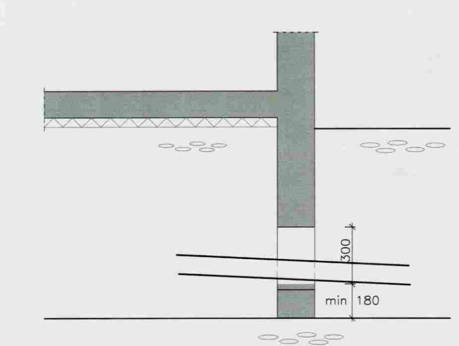
KÓTAR, SKÝRINGAR 1:20
