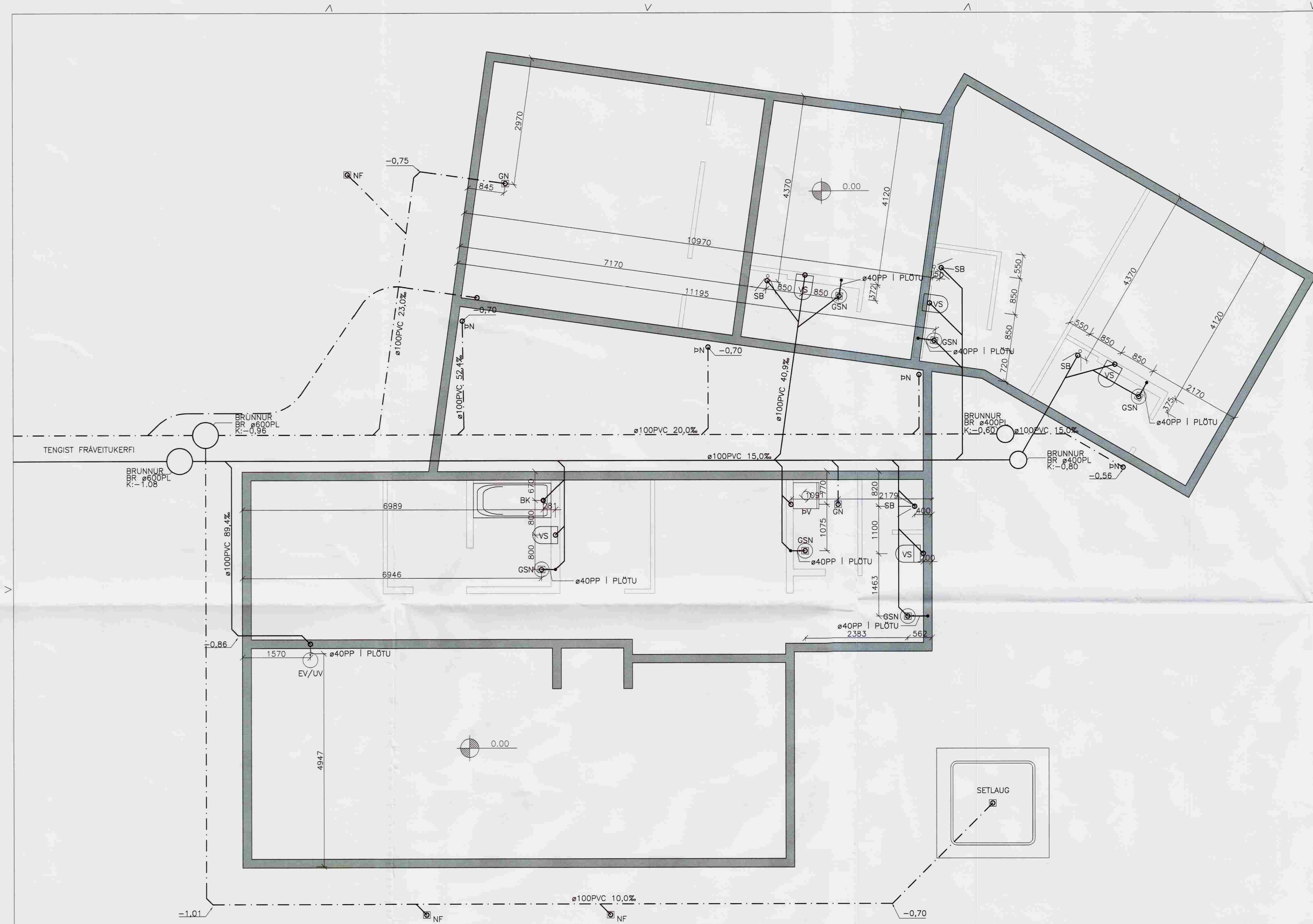
GRUNNMYND FRÆRENNSLAGNIR 1:50
