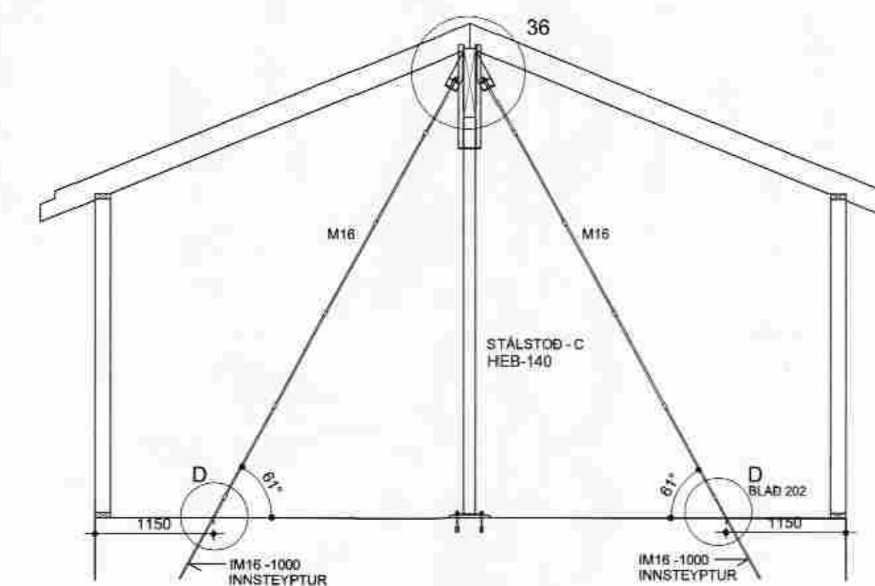
ÞVERSNIÐ N-N 1:50
