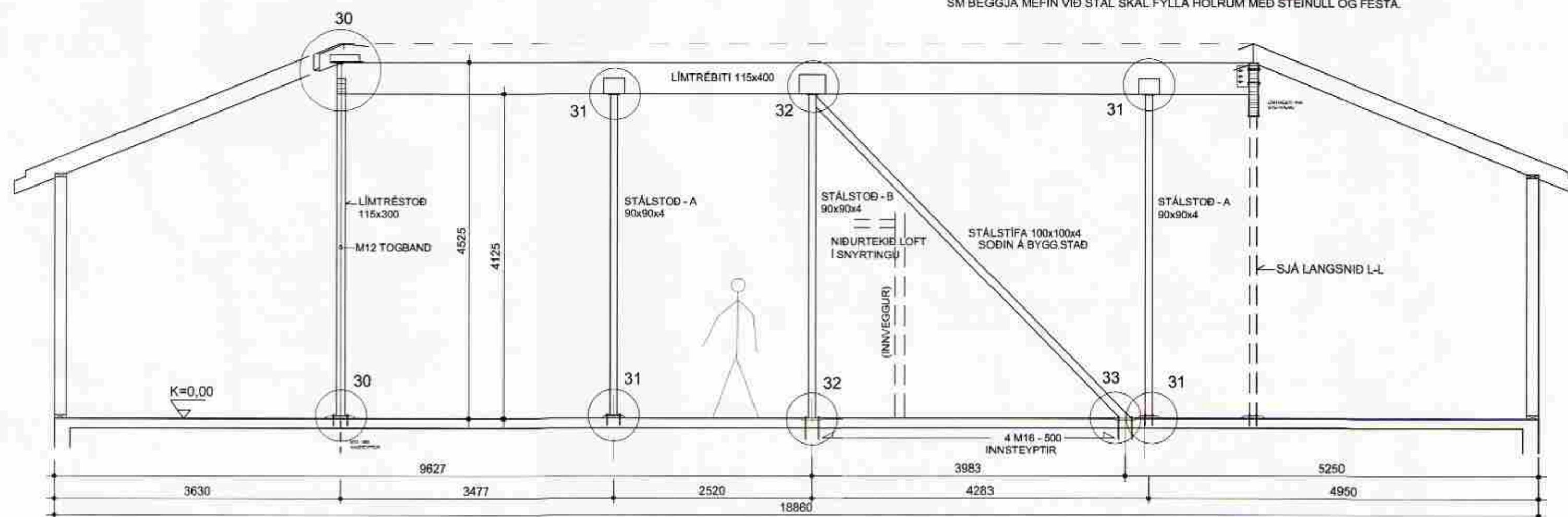
LANGSNID M-M 1:50
