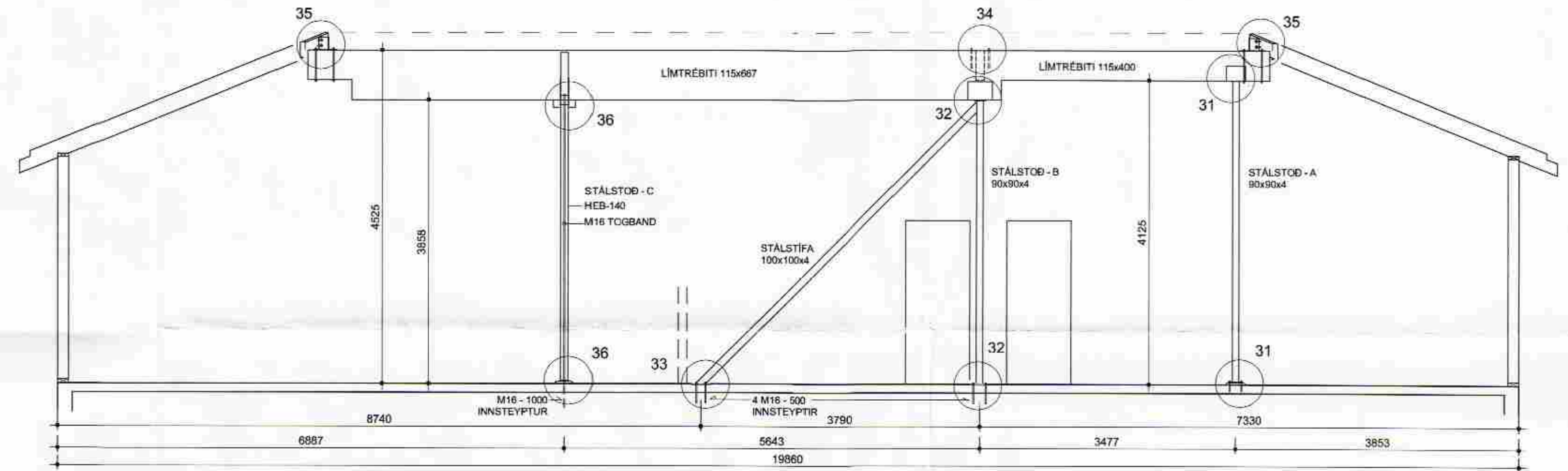
LANGSNID L-L 1:50
