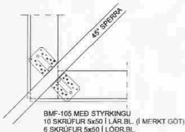
SNID A-A
