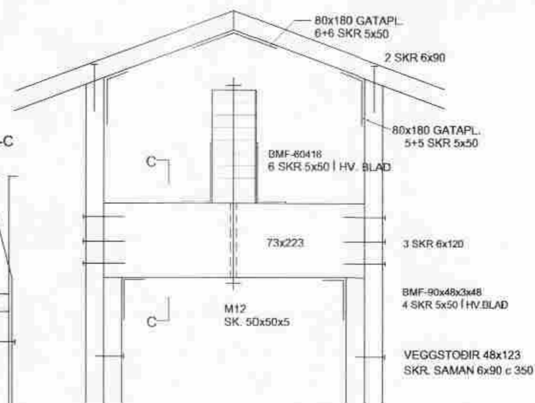
DEILI 30 1:10
