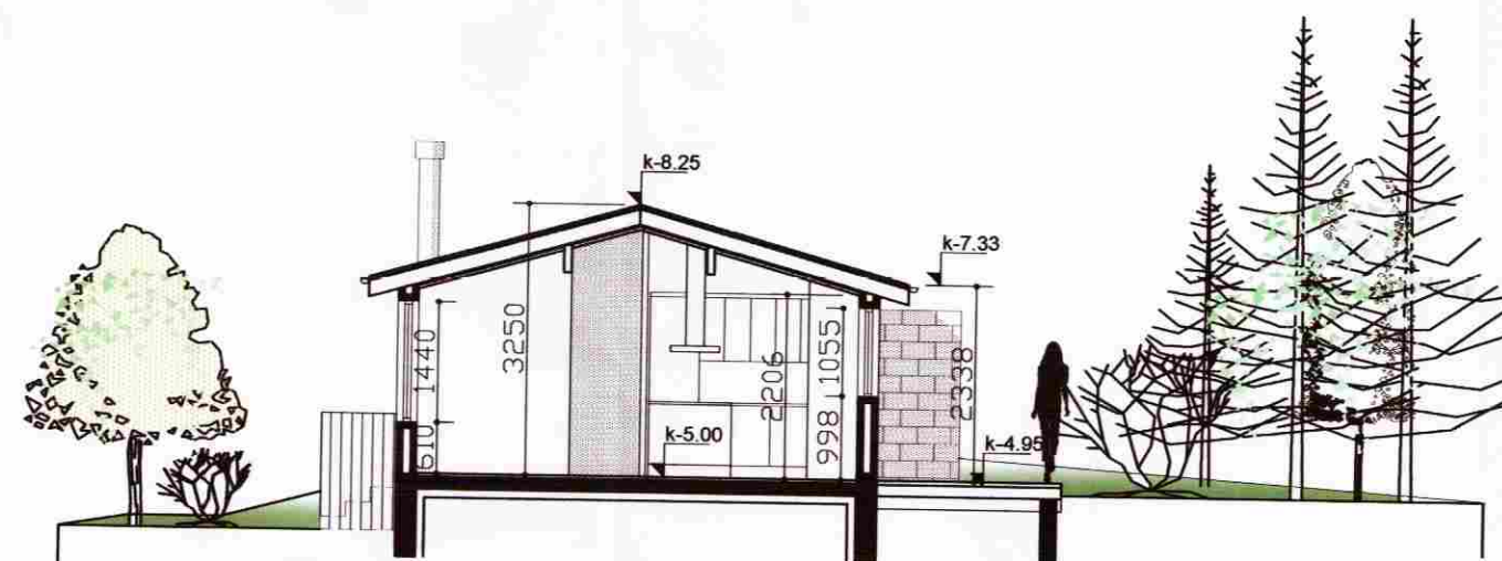
SNIÐMYND A-A. mkv. 1.100
