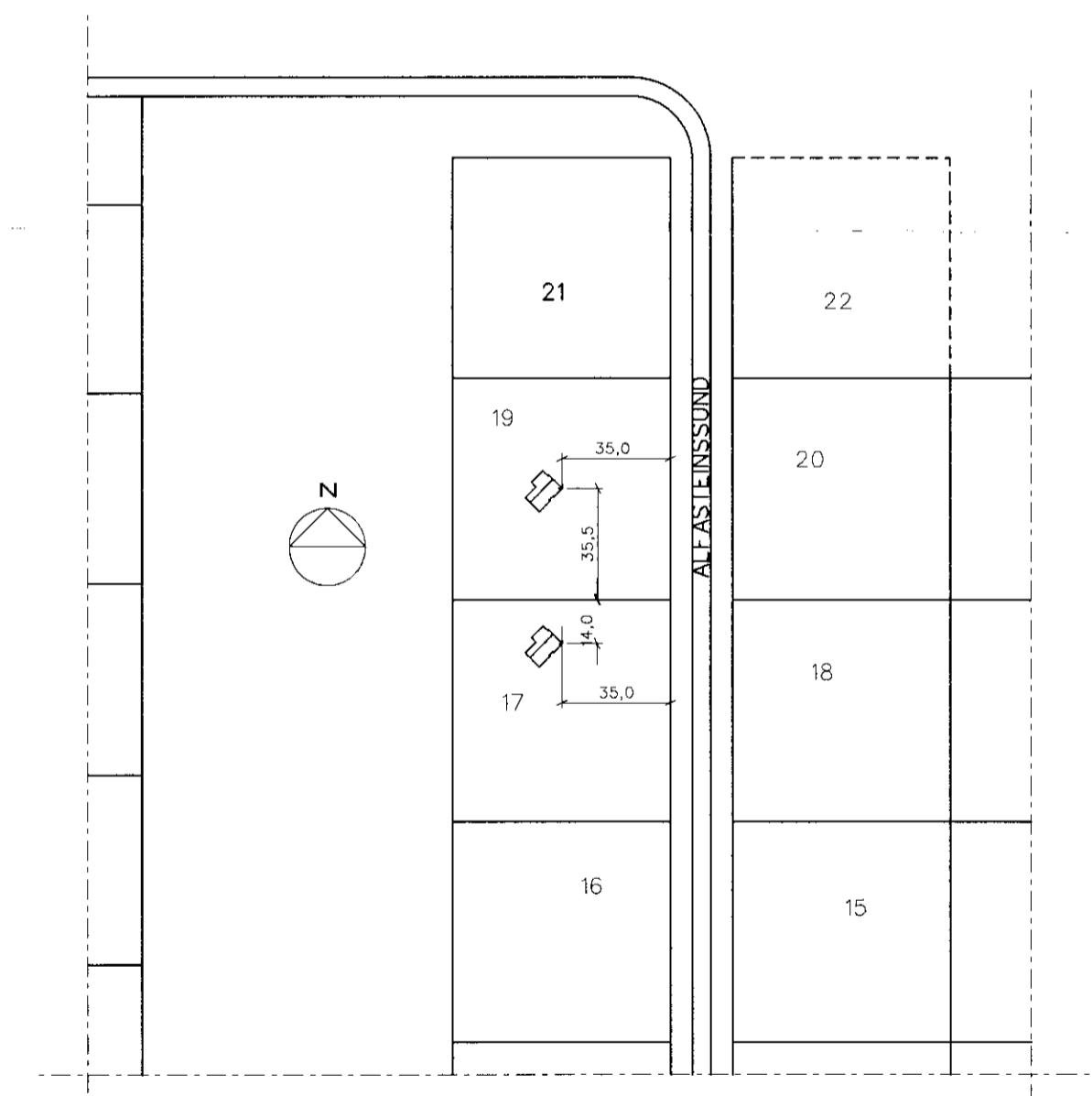
AFSTÖÐUMYND 1:1000
