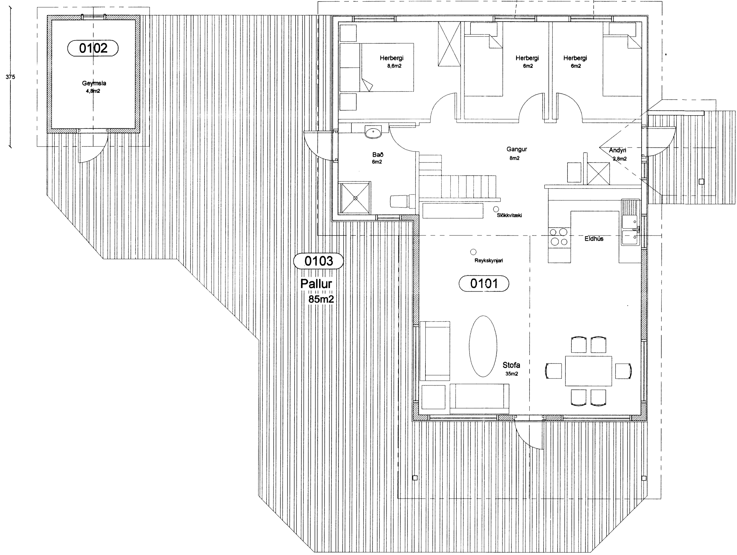
Grunnmynd (pallur) Mælikvarði 1:50
