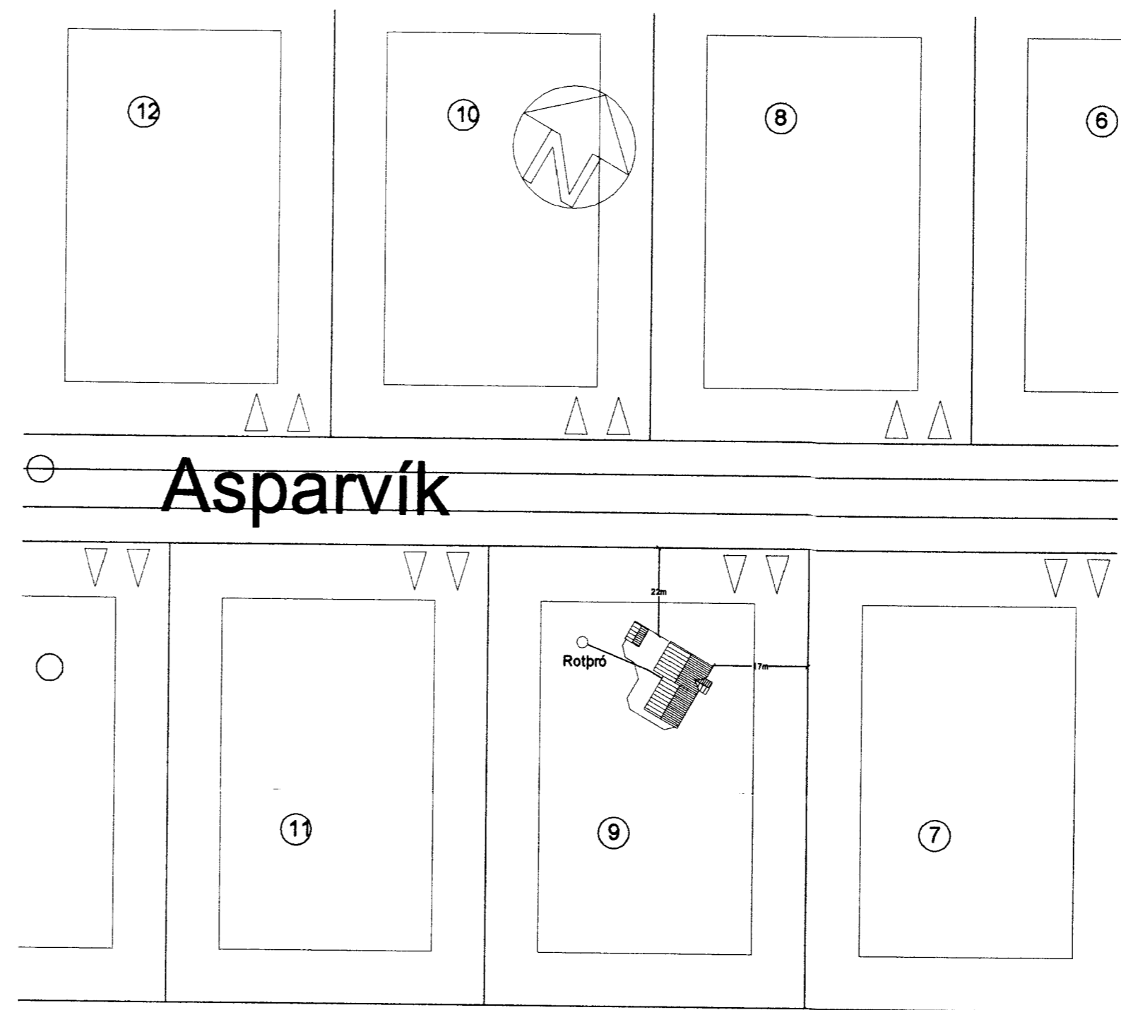
Útlit Suður Mælikvarði 1:100
