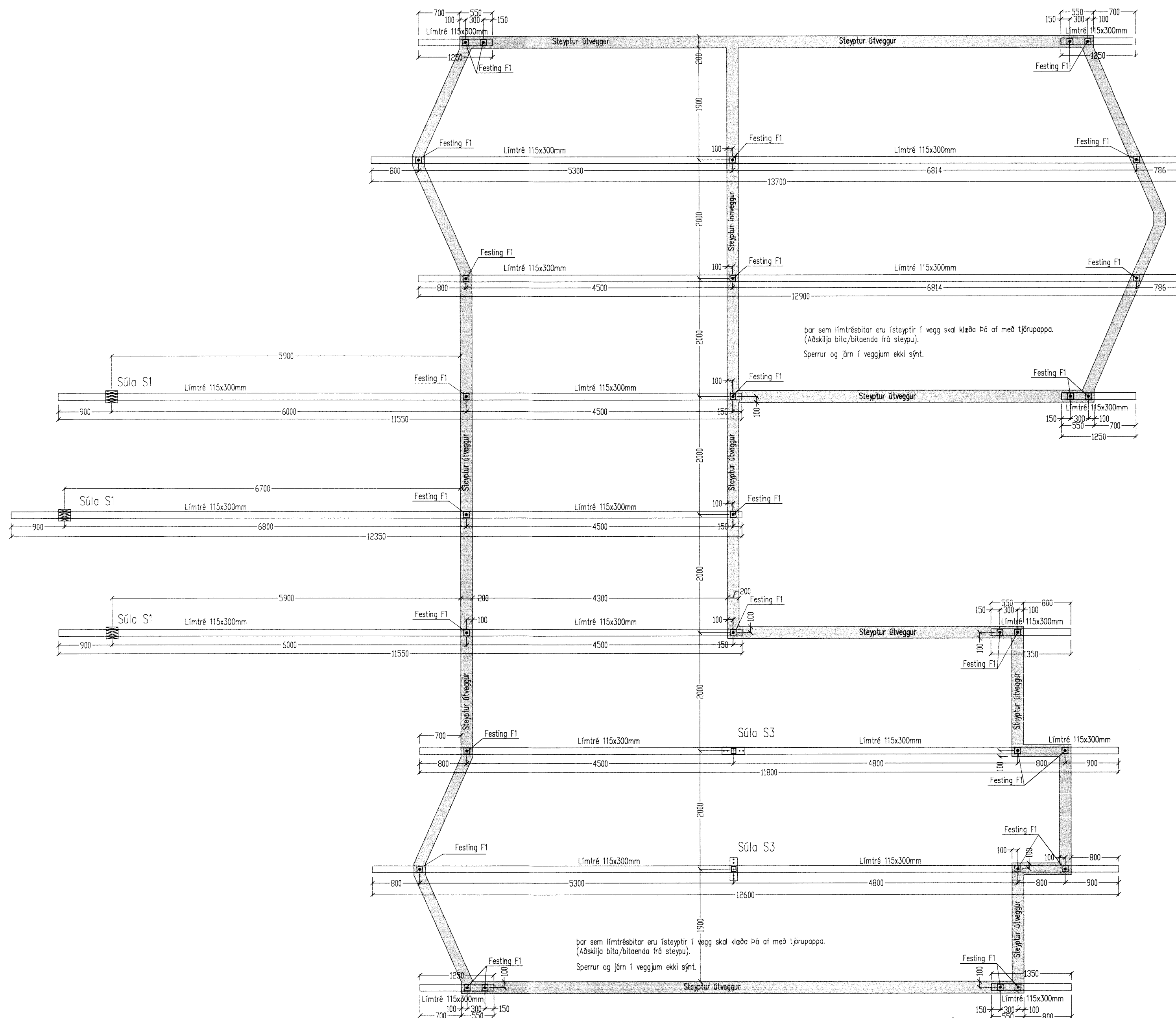
Grunnmynd límrésbita í þaki 1:50
