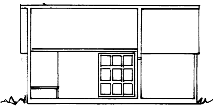
SKURÐUR B-B
