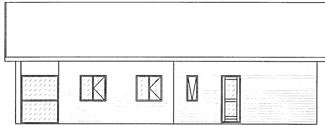
Útlit suðaustur 1:100
