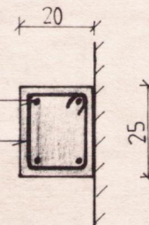
SNID í STÖÐ „S“ M = 1:20
