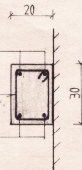
SNID í STÖÐ „S“ M = 1:20
