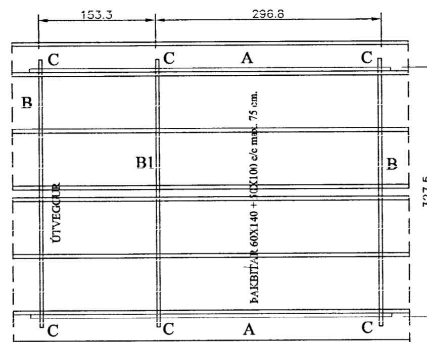
Grunnmynd þak
