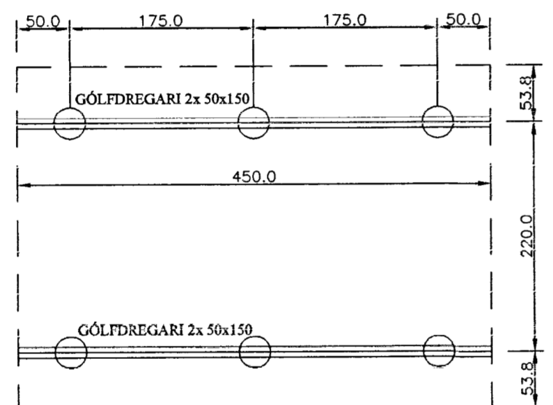
Grunnmynd dregarar
