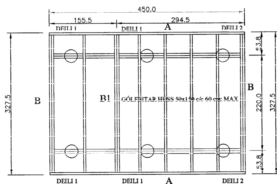
Grunnmynd gólfbitar
