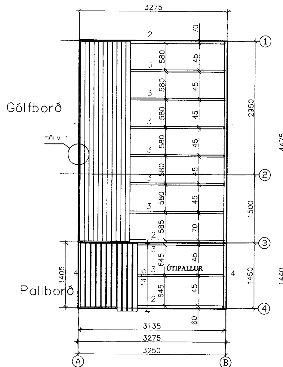
Grunnmynd gólfborð
