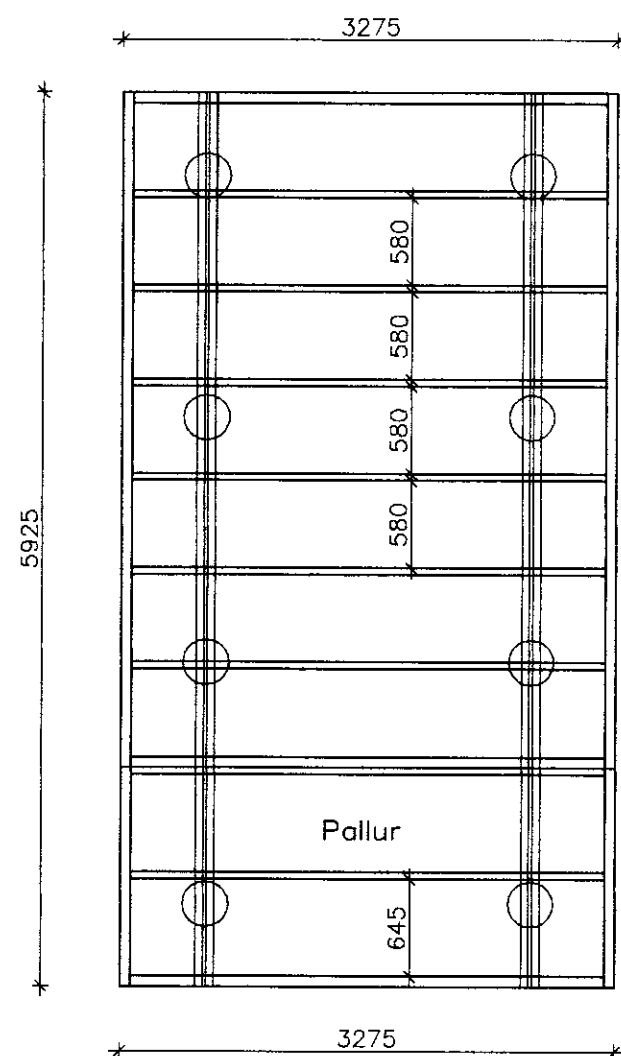
Grunnmynd dregarar
