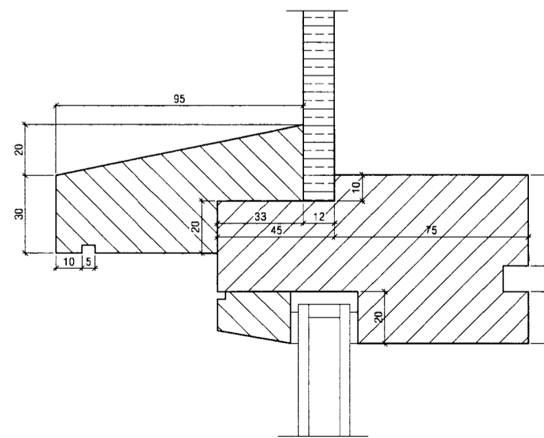
ÞVERSNIÐ KARMS/VATNSBRETTIS 1:2
