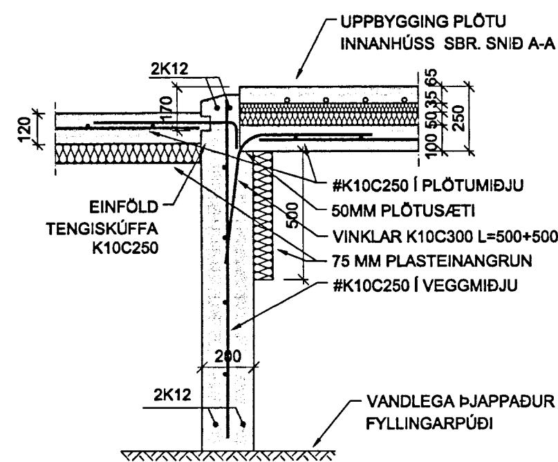
E SNEIÐING 01 Mkv. 1/20
