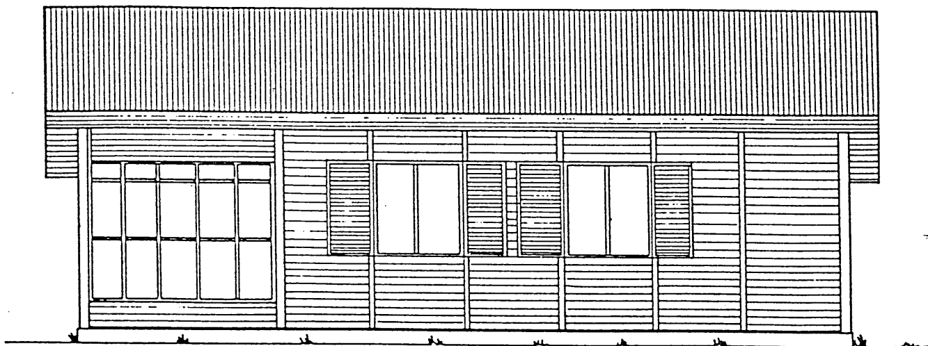
AUSTLÆG HLID 1:50
