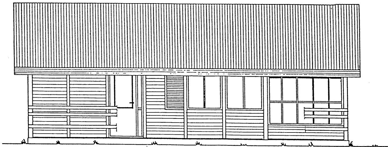
VESTLÆG HLID 1:50
