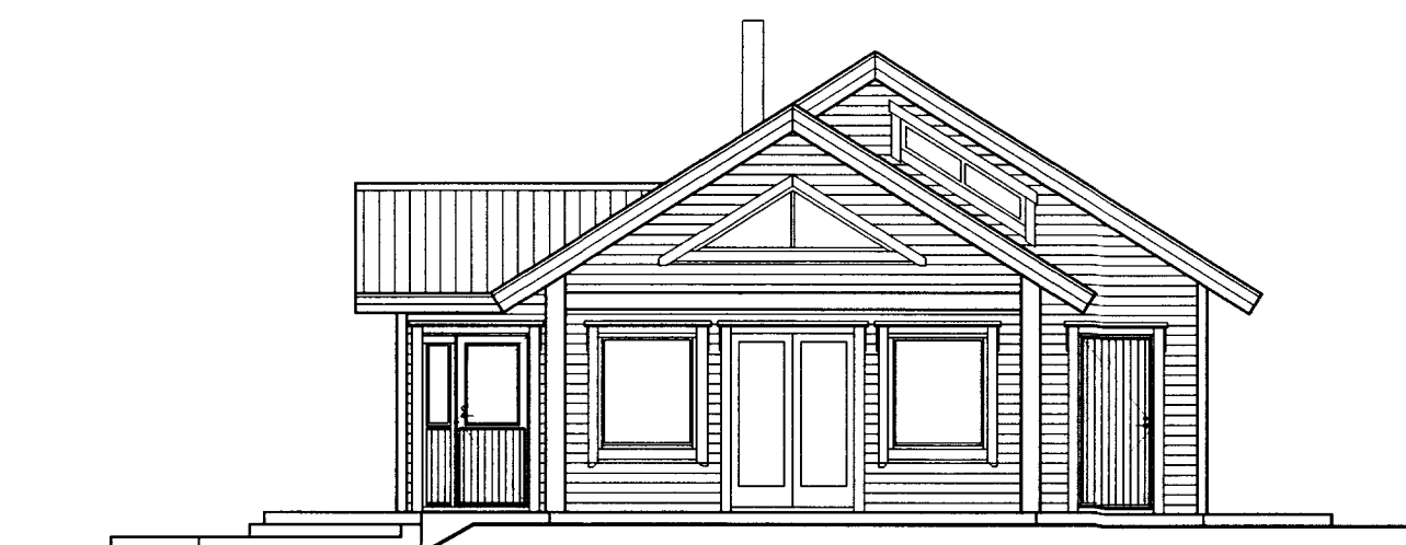
ÚTLIT SUÐVESTURHLIÐ
