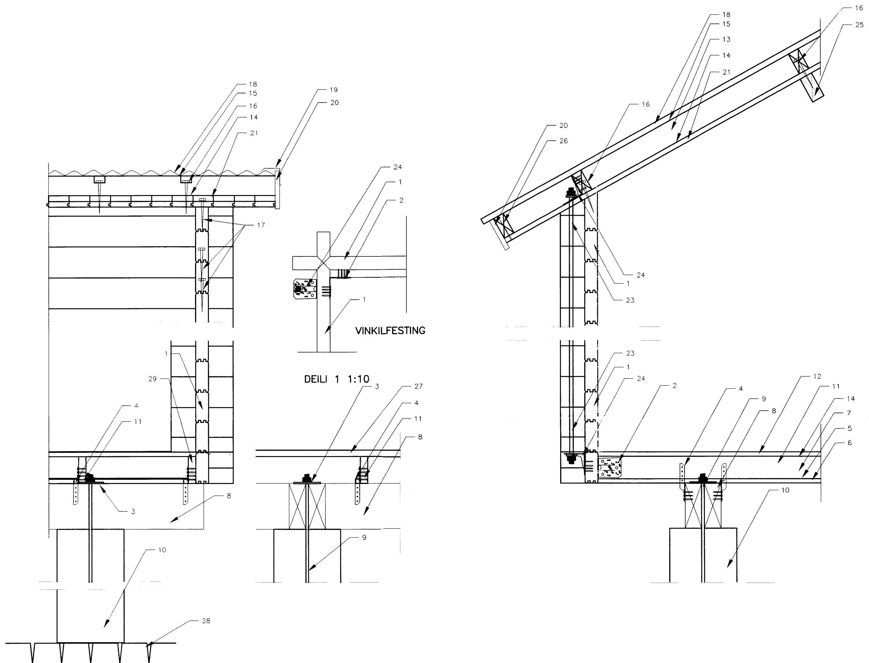
ALMENN SNID 1:10
