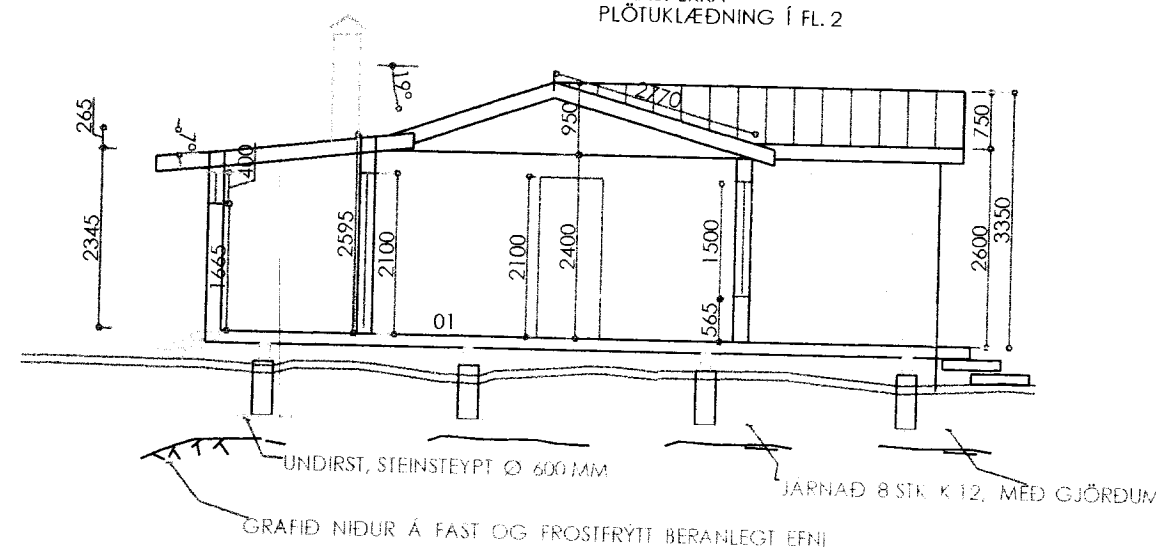
SNÍÐ A - A MKV 1 : 100
