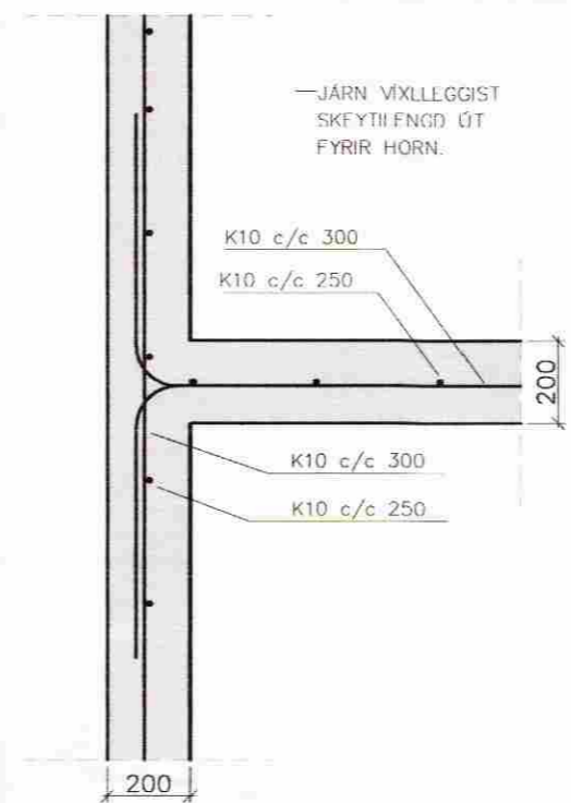
LÁRÉTT SNIÐ Í SÖKKULVEGG Mkv. 1:20
