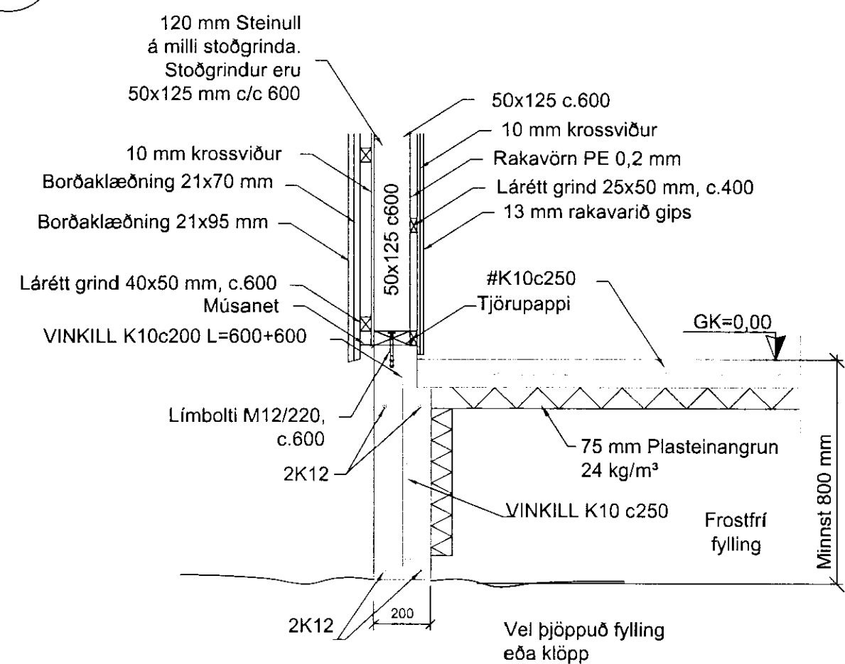
A Snið A-100 1:20
