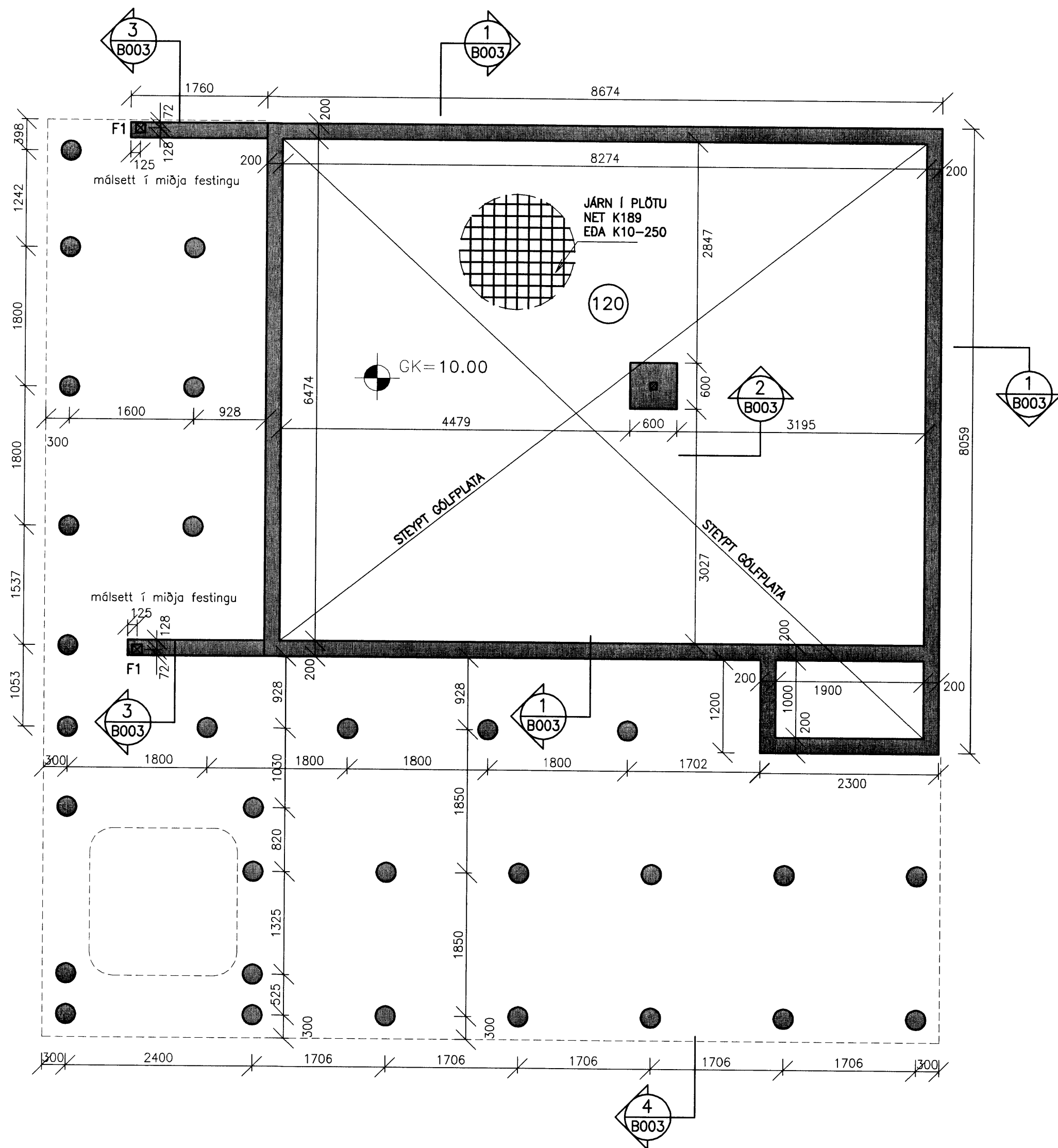
GRUNNMYND UNDIRSTÖÐUR 1:50
