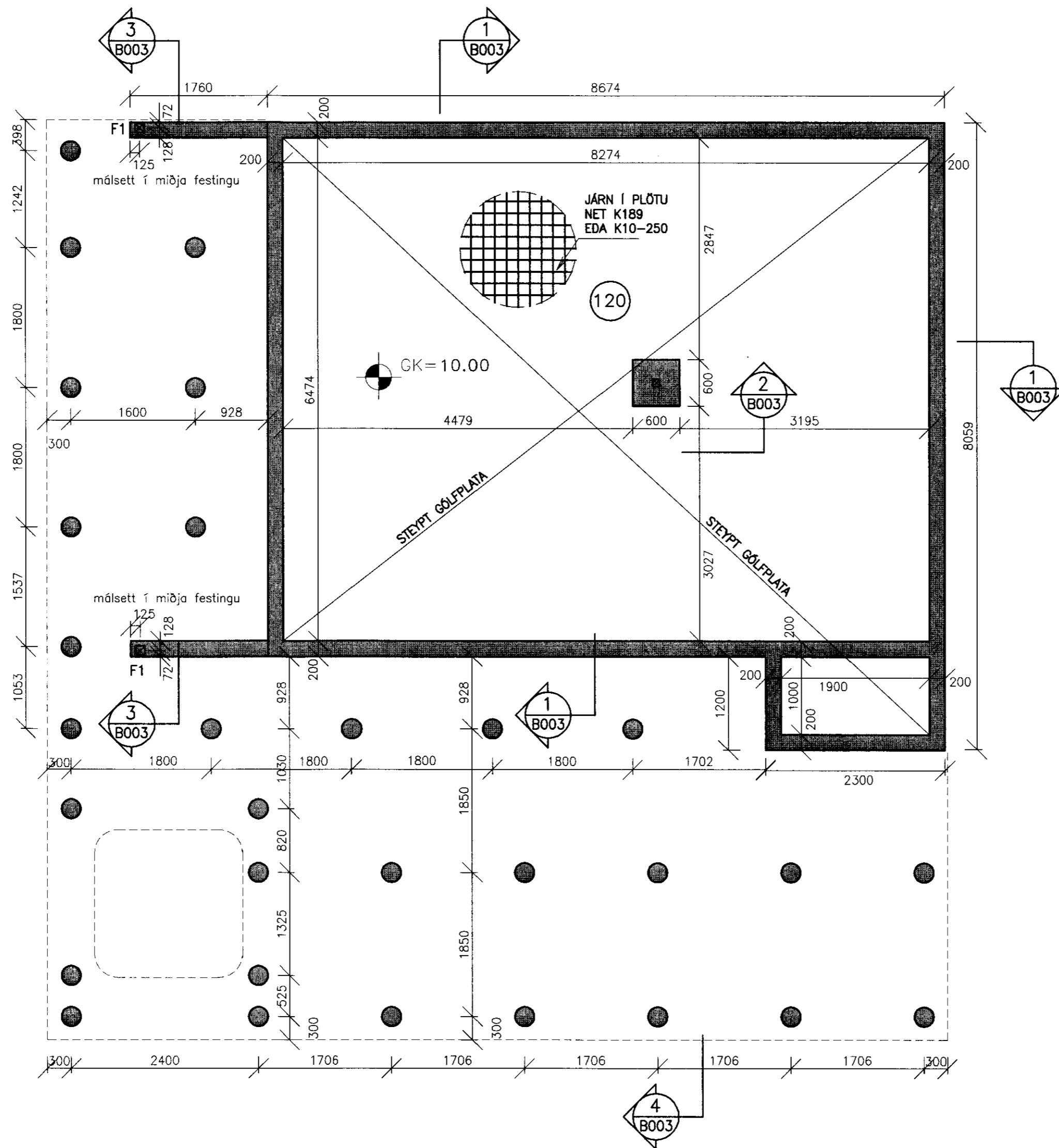
GRUNNMYND UNDIRSTÖÐUR 1:50
