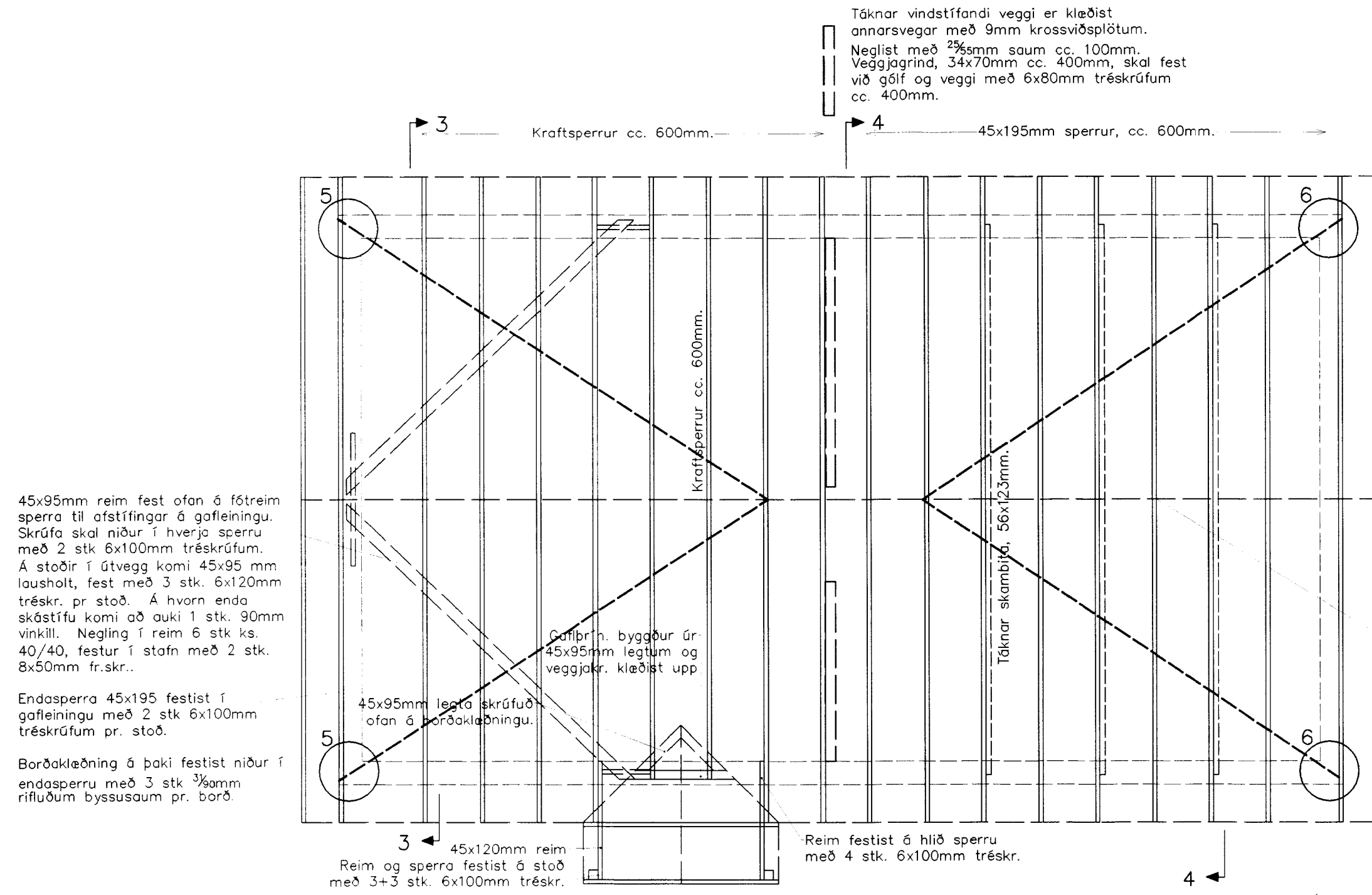
SPERRUPLAN 1:50
