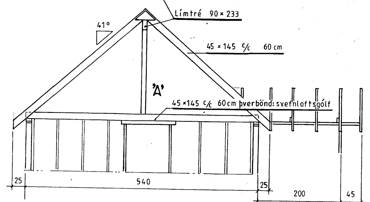
Snid A-A
