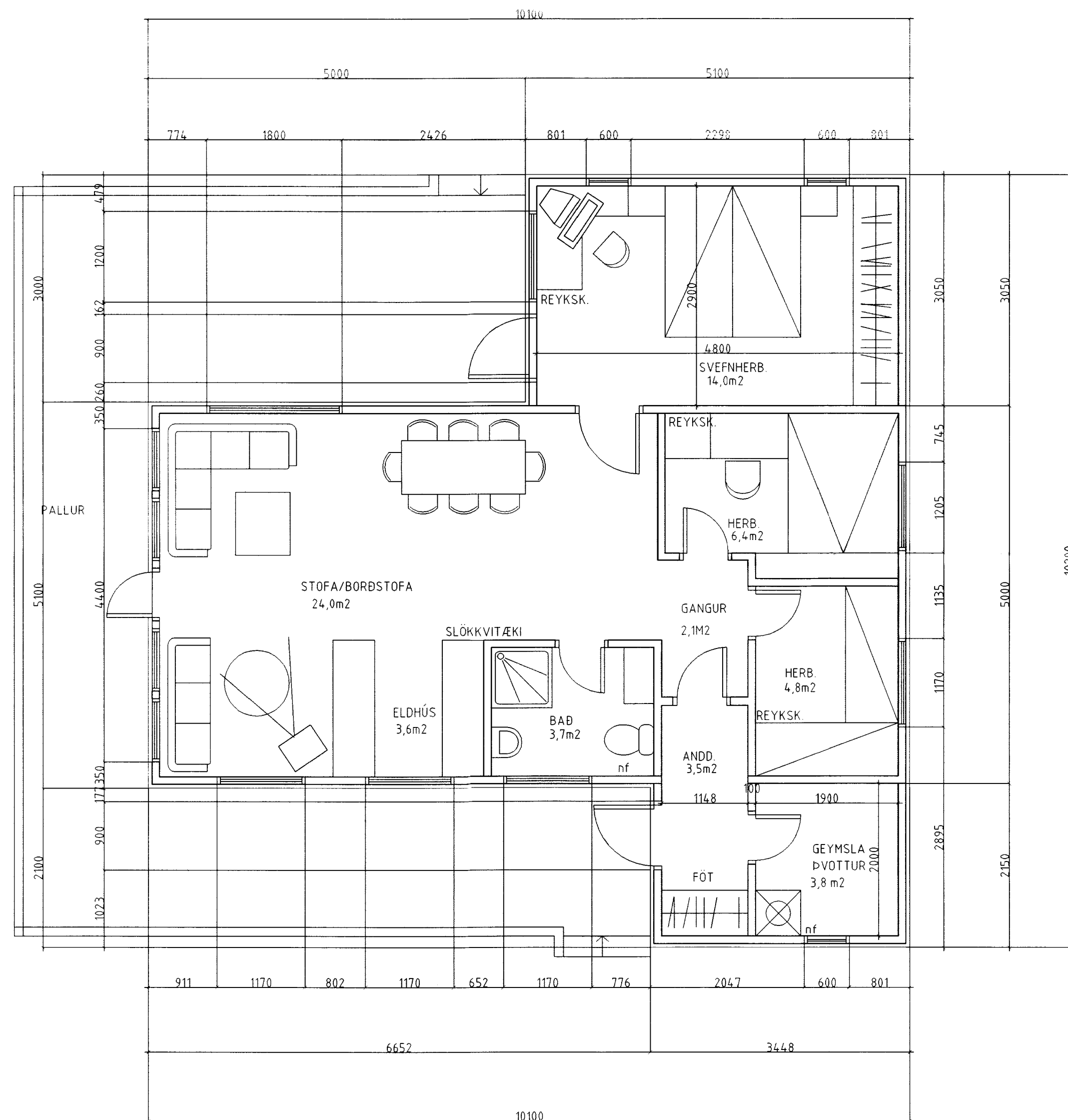
GRUNNMYND M=1/50
