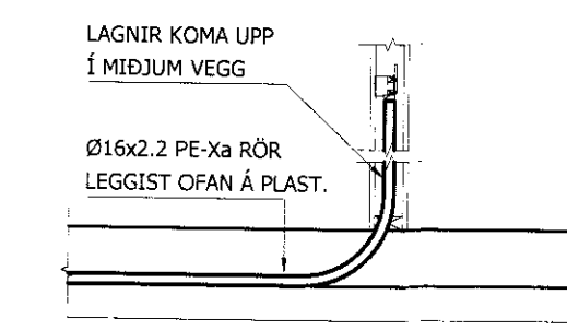
311 FRÁGANGUR NEYSLUVATNS Í MILLIVEGG Mkv 1:20
