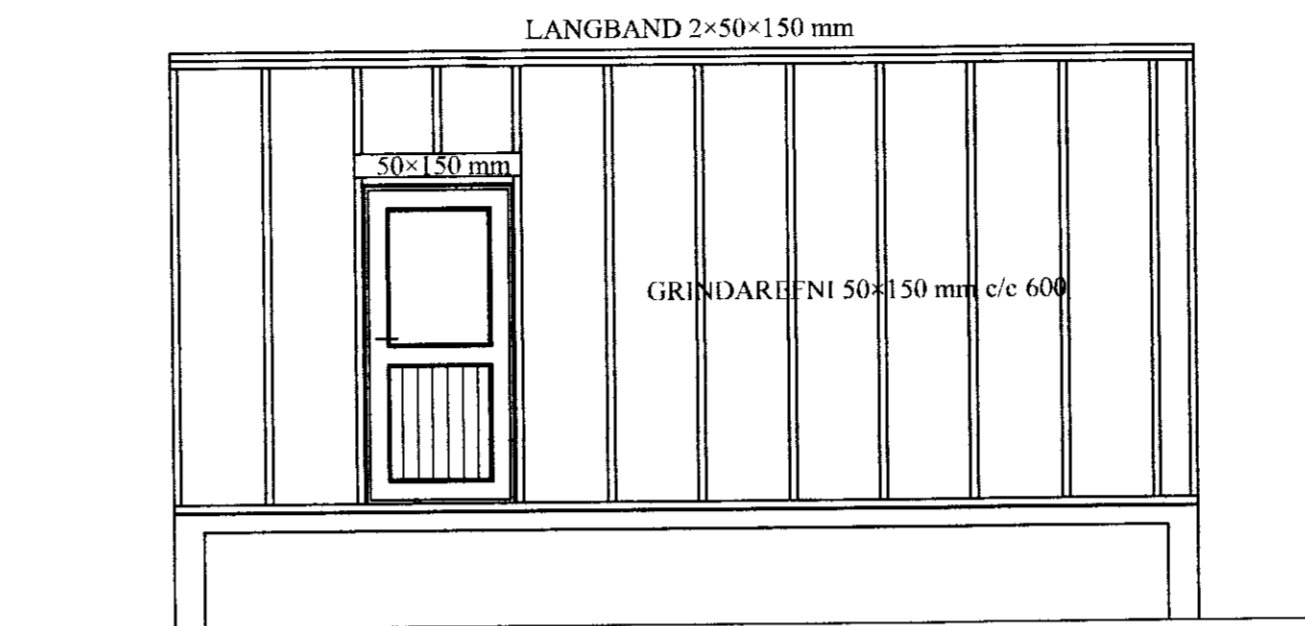
GRINDARTEIKNING AUSTURHLIÐAR
