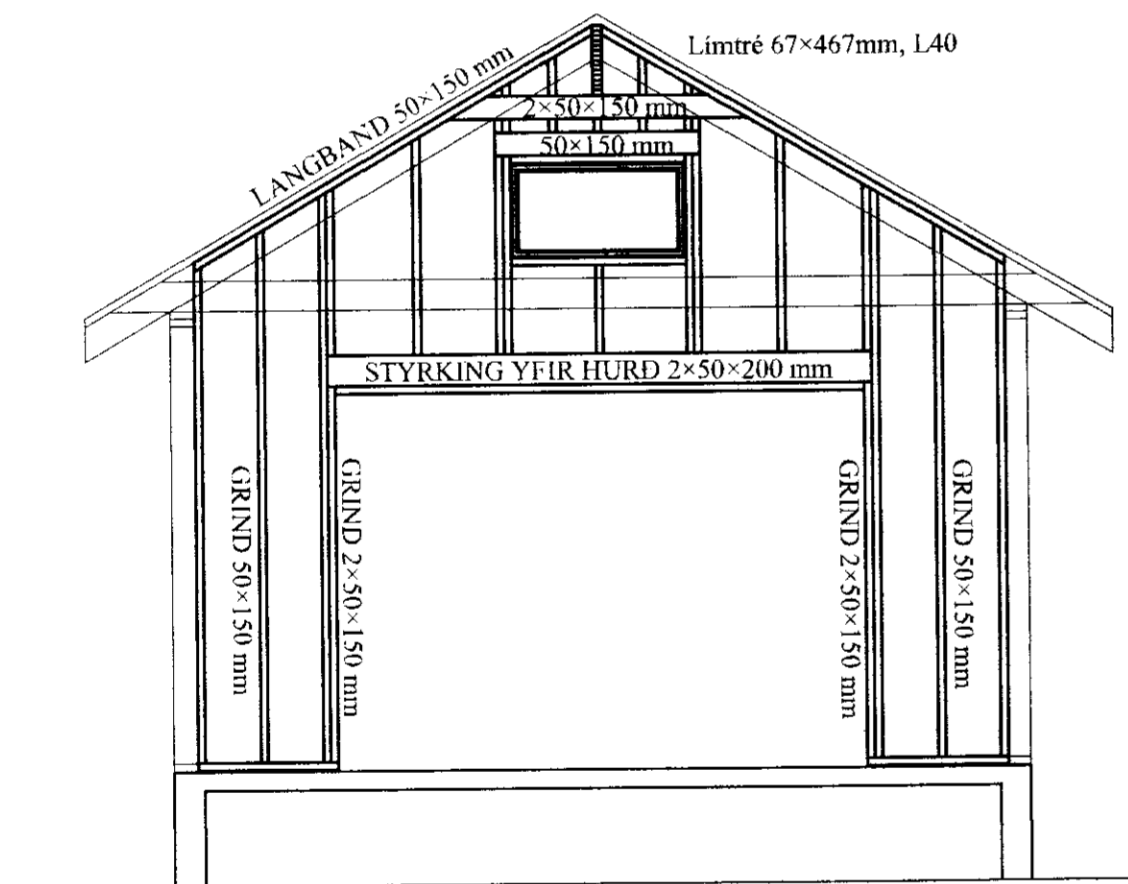
GRINDARTEIKNING NORÐURHLIÐAR
