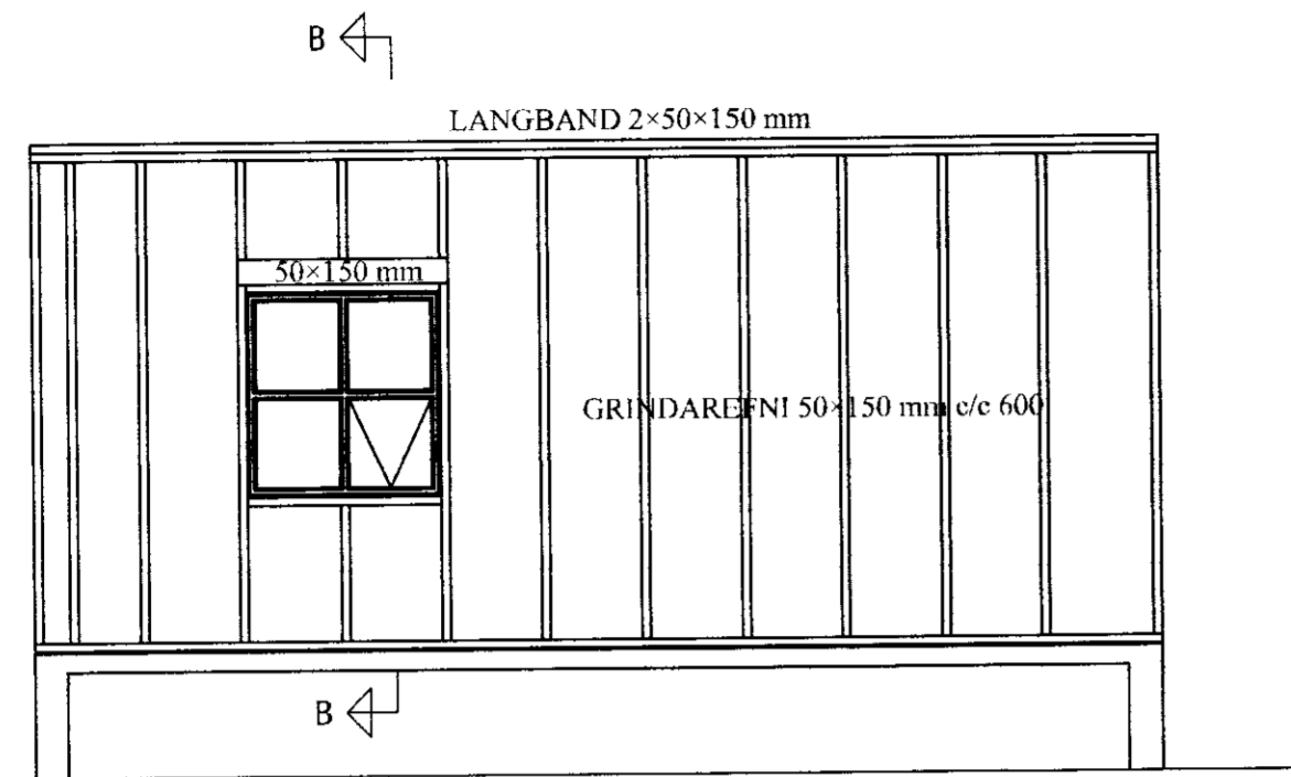
GRINDARTEIKNING VESTURHLIÐAR
