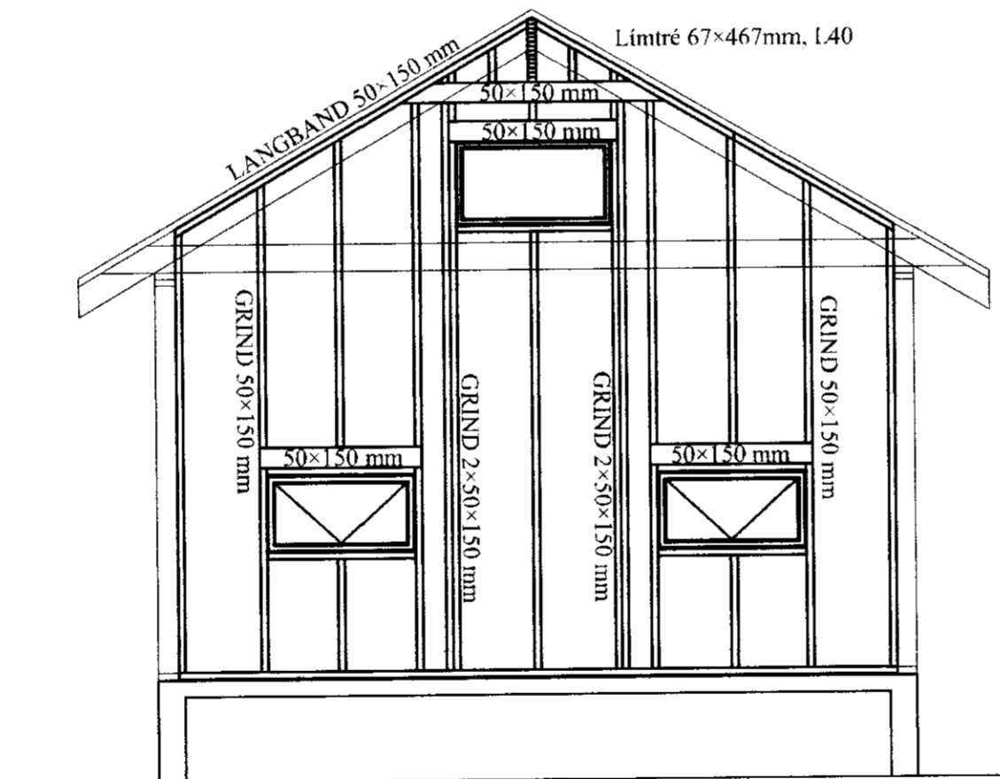
GRINDARTEIKNING SUÐURHLIÐAR
