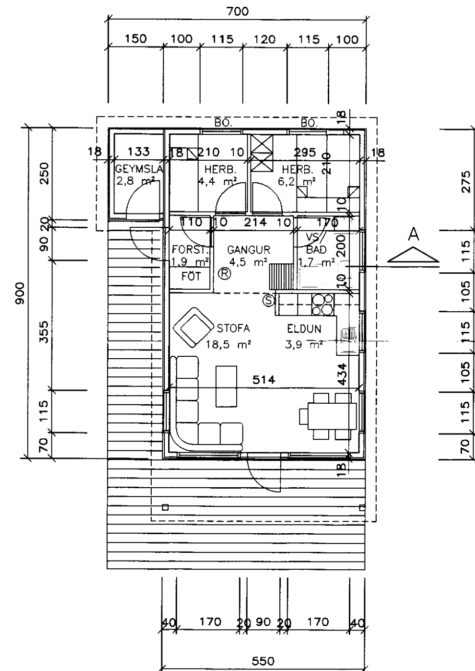
GRUNNMYND mkv. 1:100
