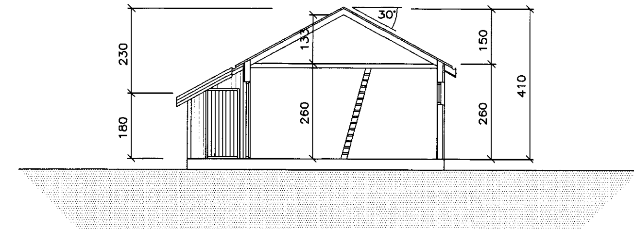
SKURÐUR A
