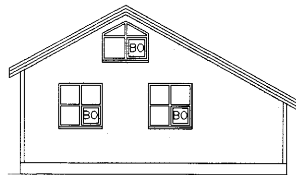
ÚTLIT NORÐ VESTUR
