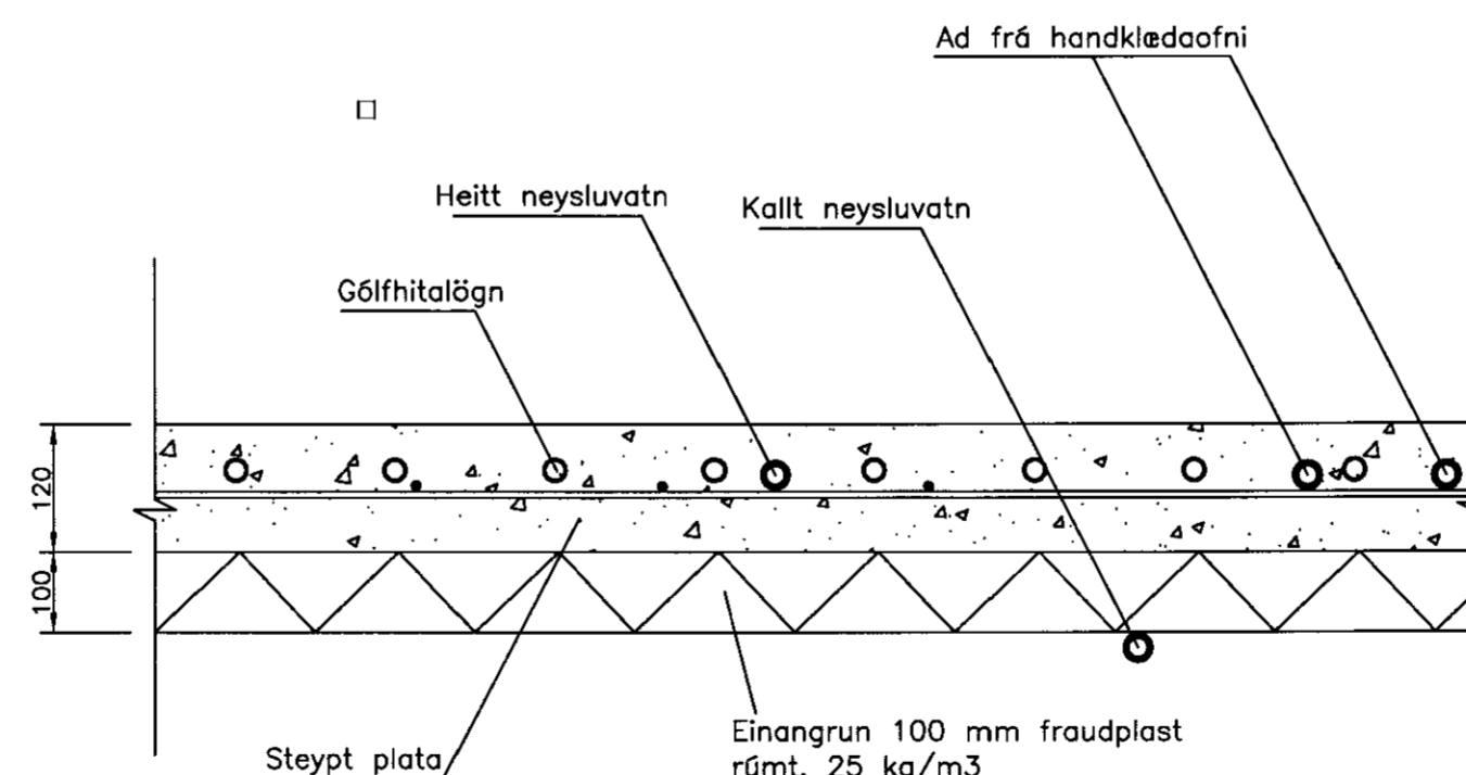
STADSETNING HITA OG VATNSLAGNA Í BOTNPLÖTU ÍBÚÐARHLUTA
