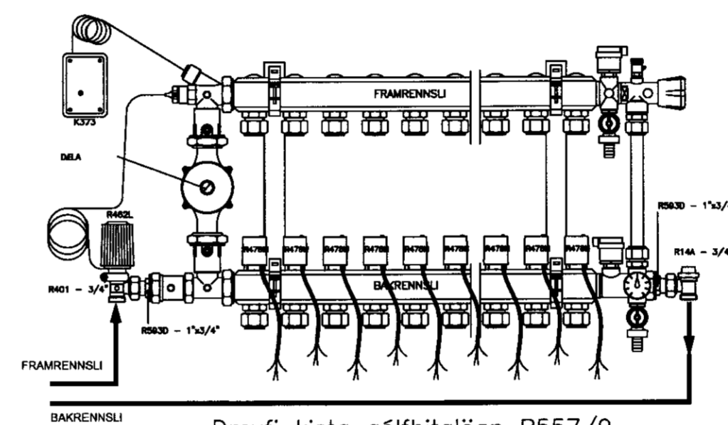
( SKEMATISK MYND )
