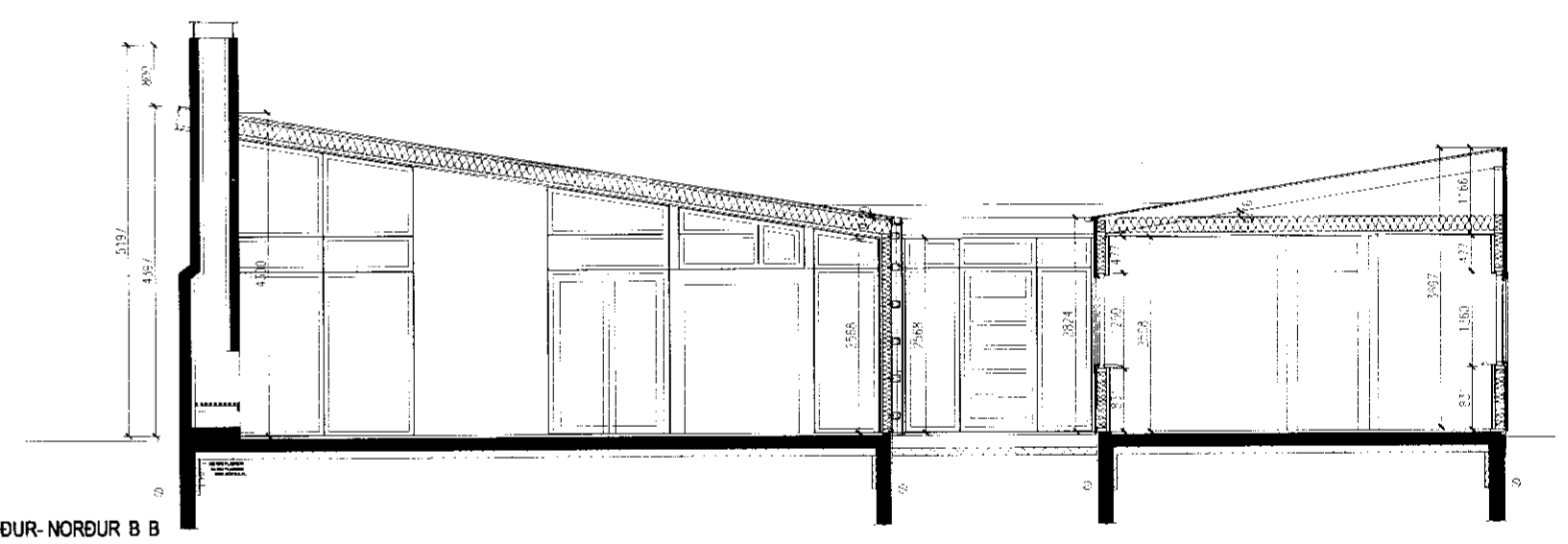
SKURÐUR SUÐUR - NORÐUR B B
