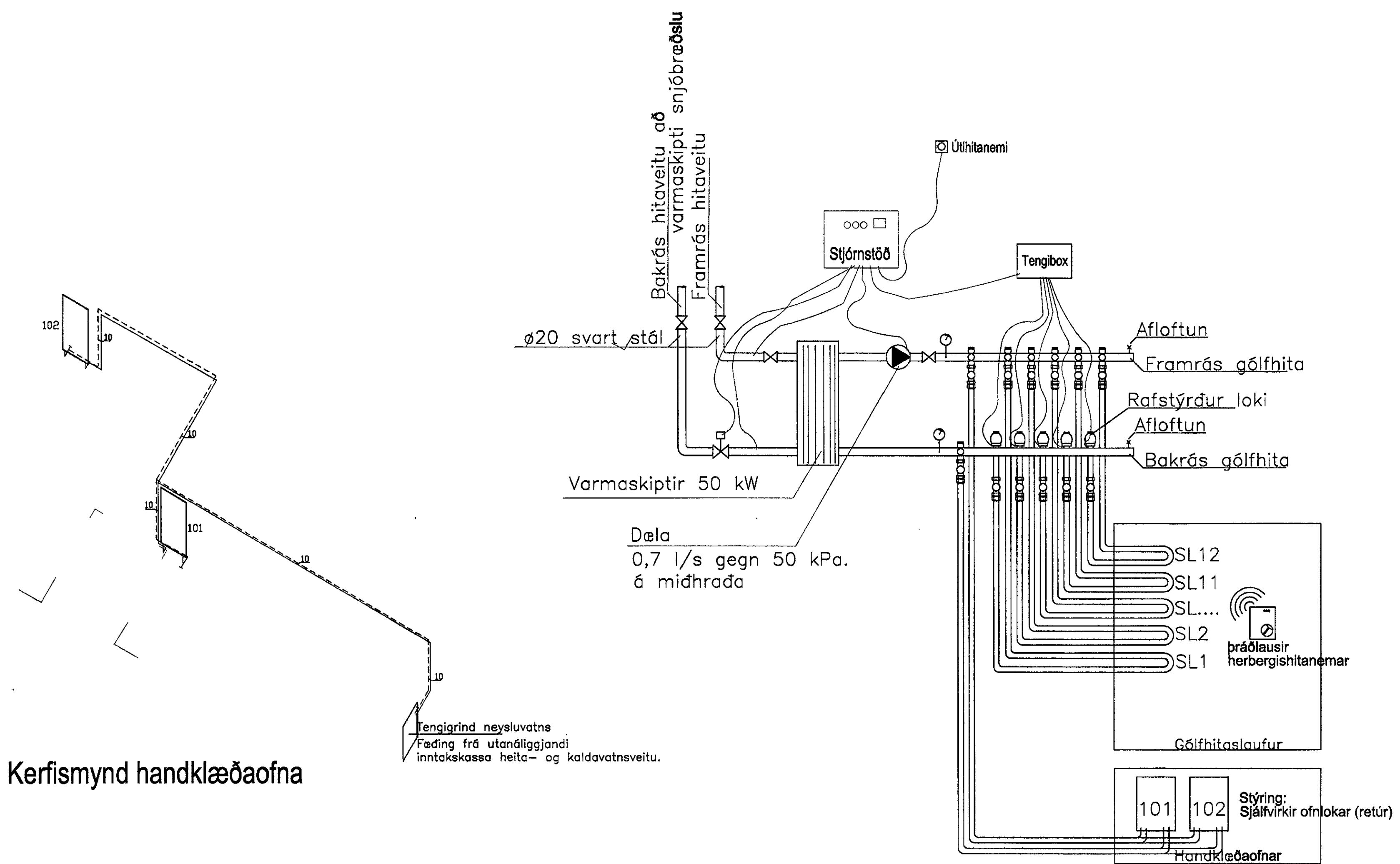
Tengigrind gólfhita / ofna í þvottahúsi (skematísk)
