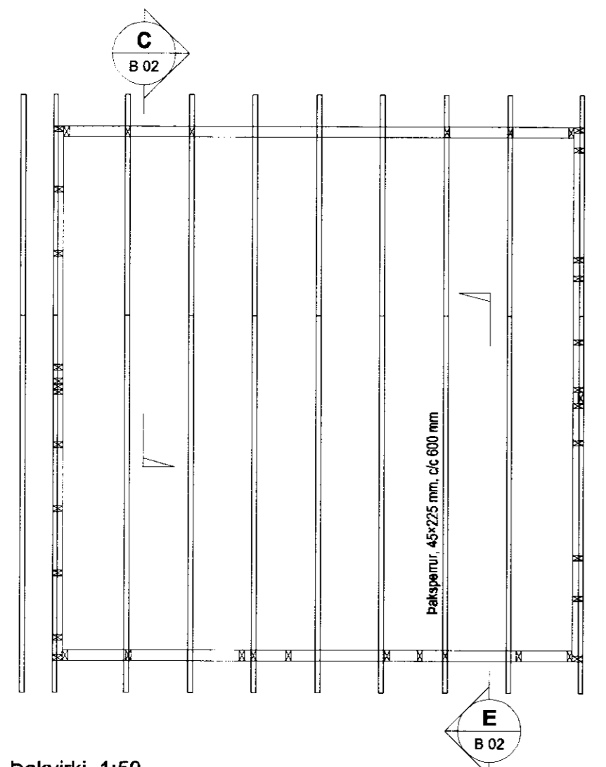
Bakvirki 1:50
