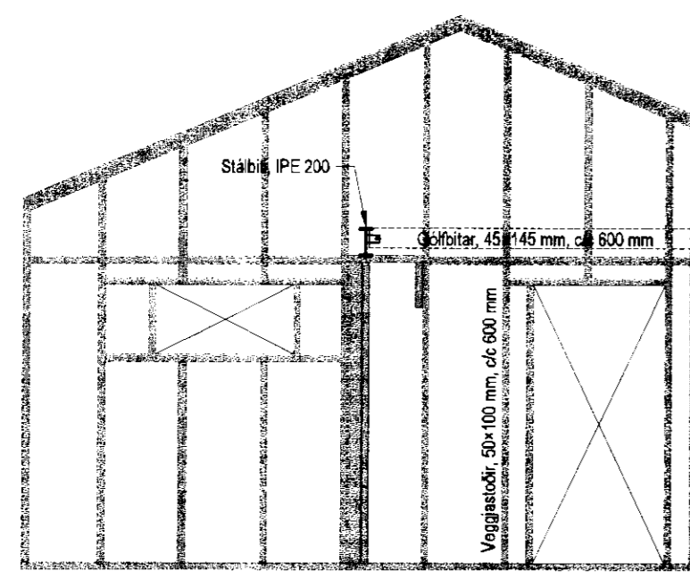
Veggjagrind, austur 1:50
