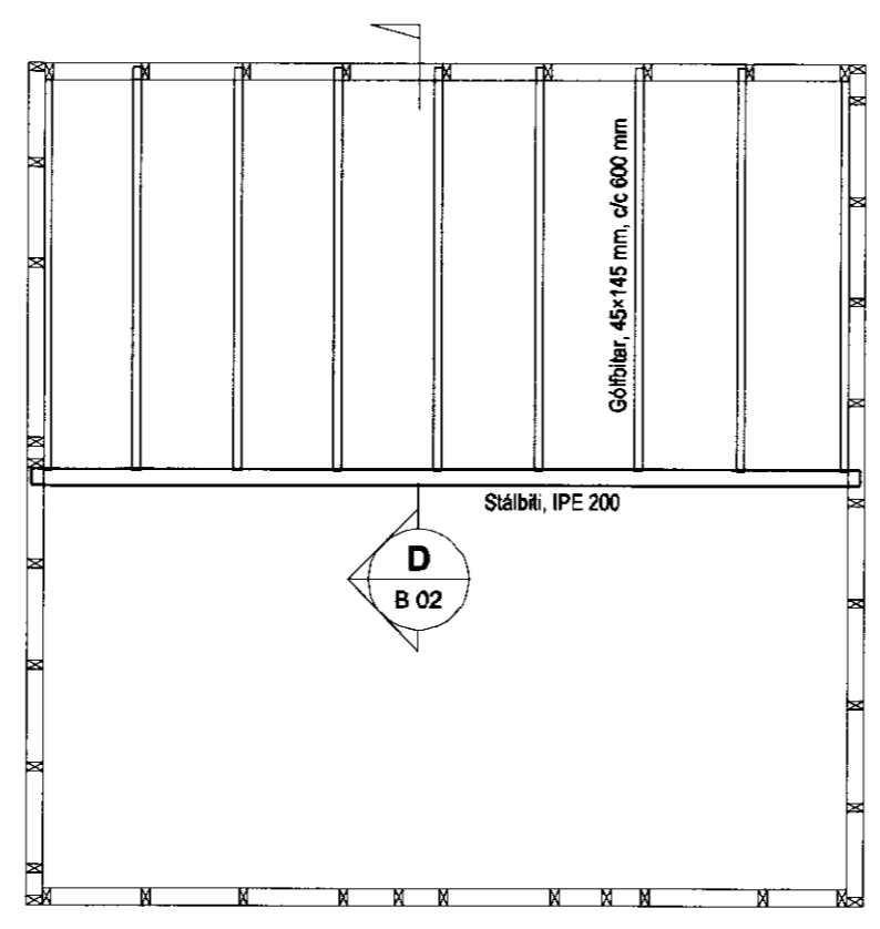
Milligólf 1:50
