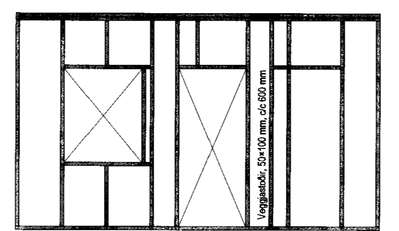
Veggjagrind, suður 1:50
