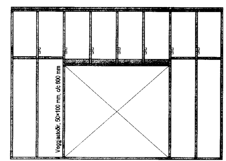
Veggjagrind, norður 1:50
