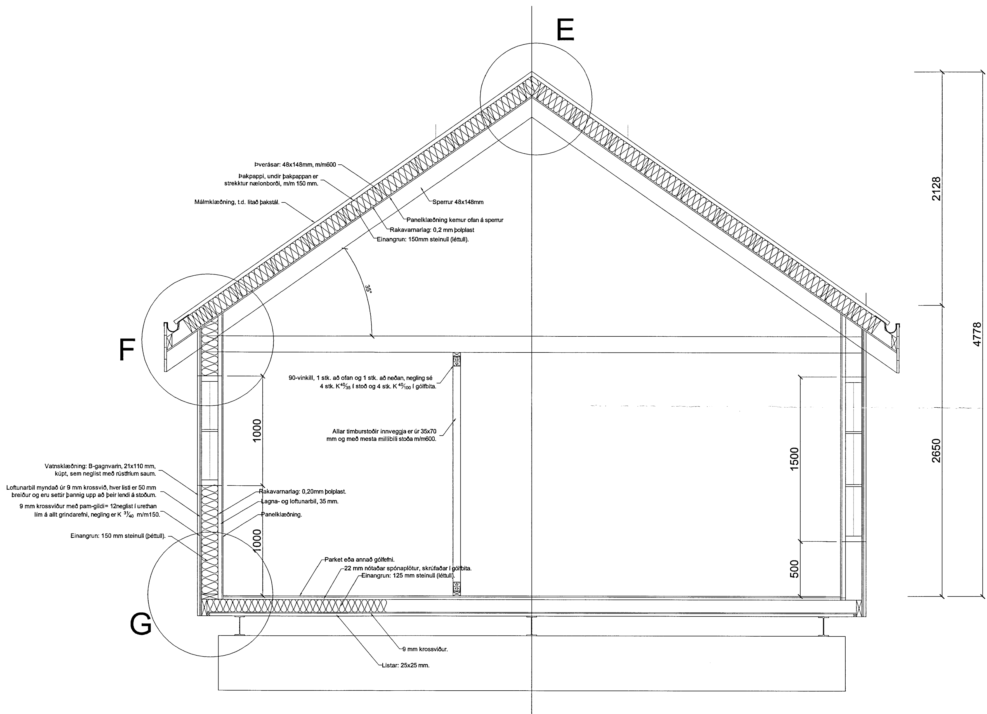
Þversnið í sumarhús með efnisskýringum.
