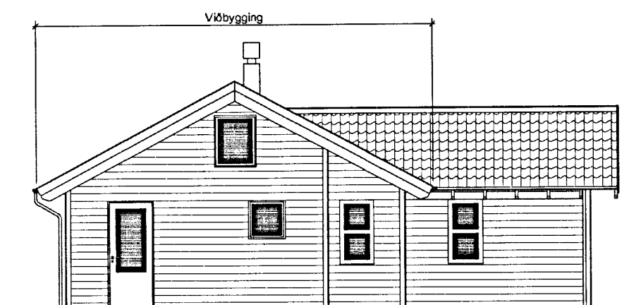
ÚTLIT NORDUR 1:100
