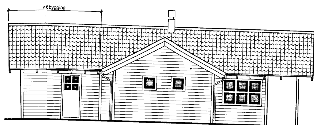
ÚTLIT VESTR 1:100
