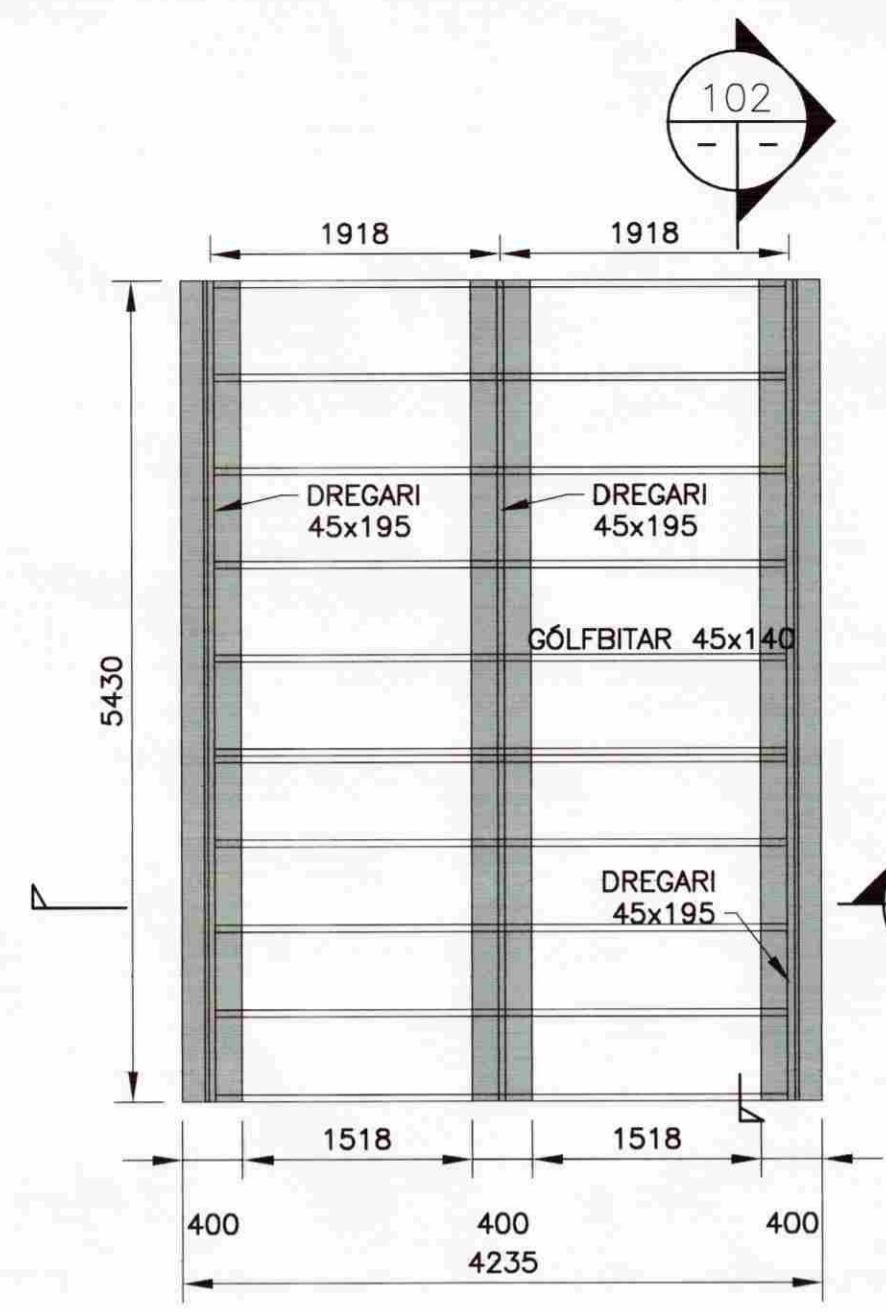
GRUNNMYND-UNDRISTÖÐUR MKV. 1
