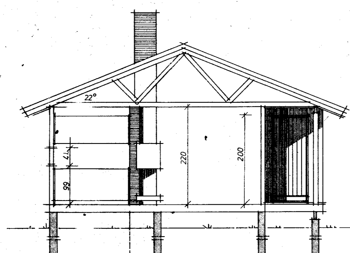
FUNDAMENTERES TIL FJELL ELLER FROSTFRI DYBDE
