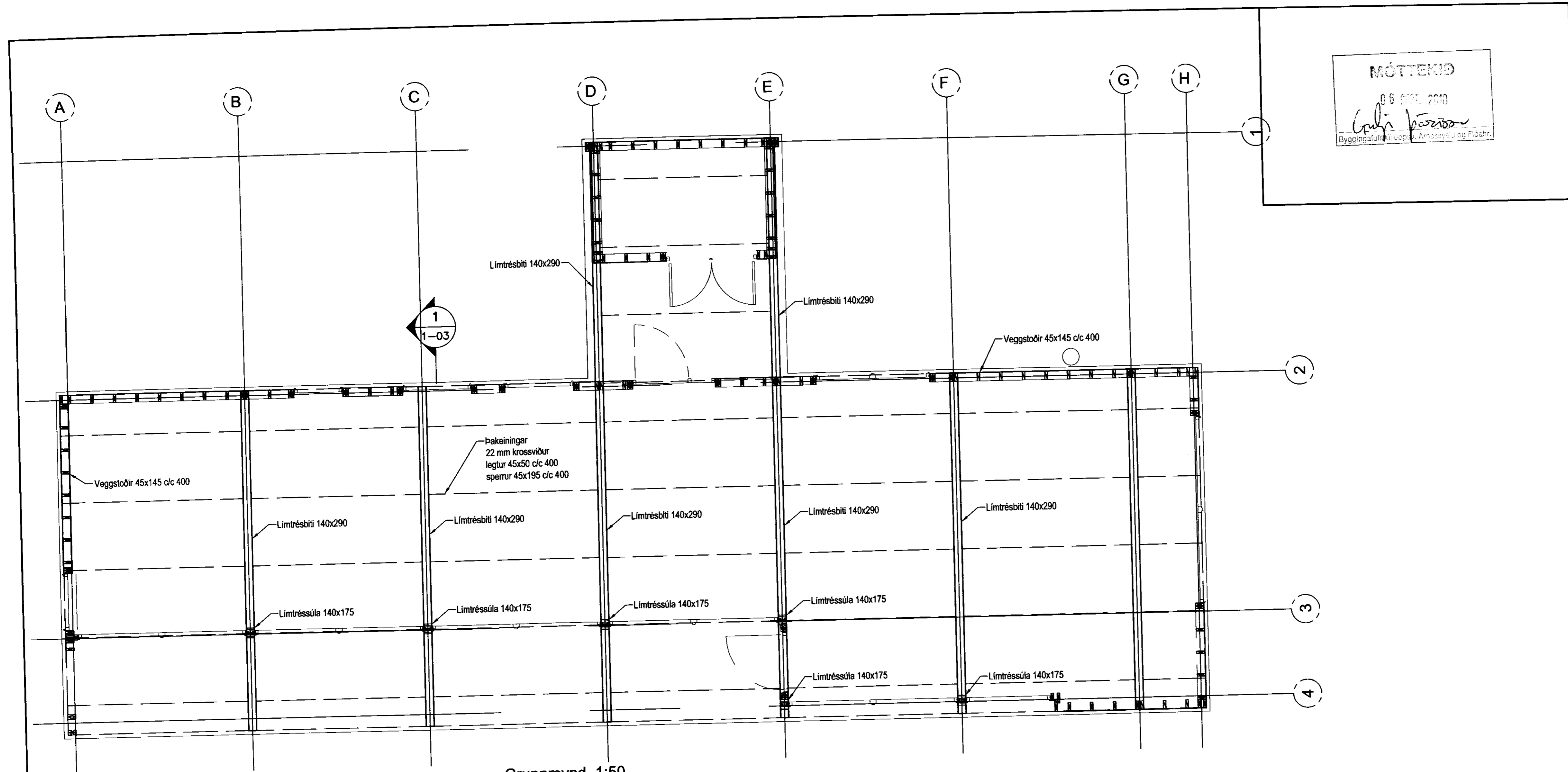
Grunnmynd, 1:50
