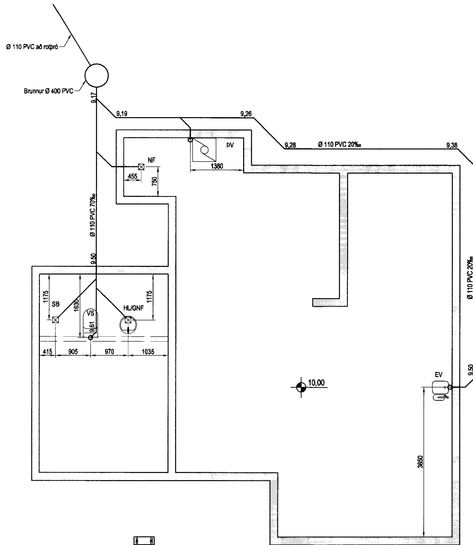
Grunnlagnir, Grunnmynd, 1:50
