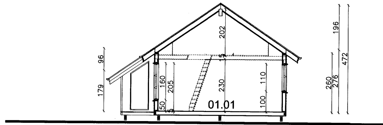
SKURÐUR A.
