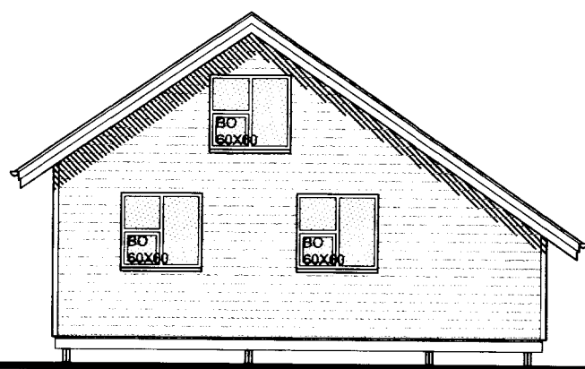
ÚTLIT NORÐUR
