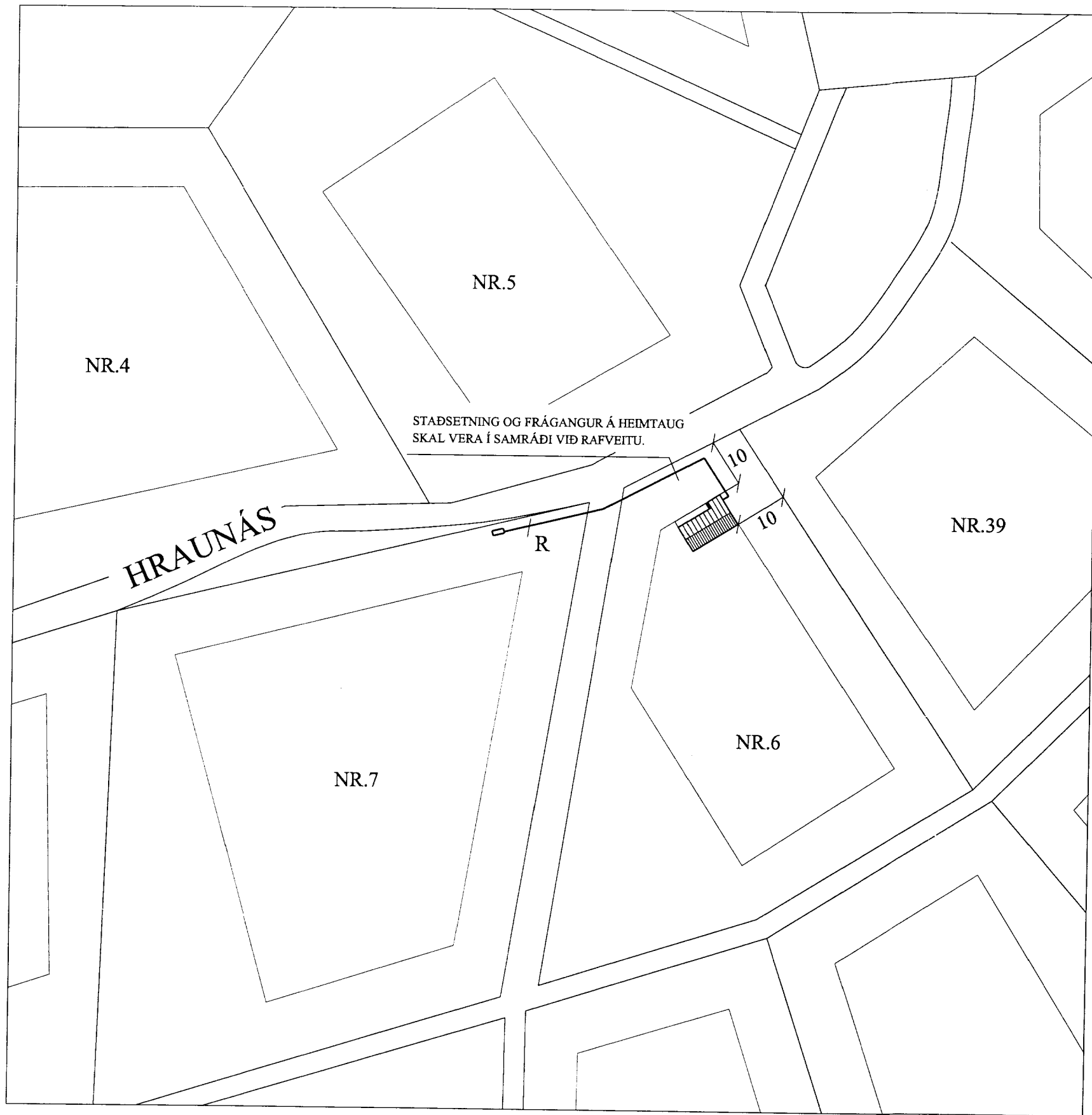
AFSTÖÐUMYND MKV. 1:1000
